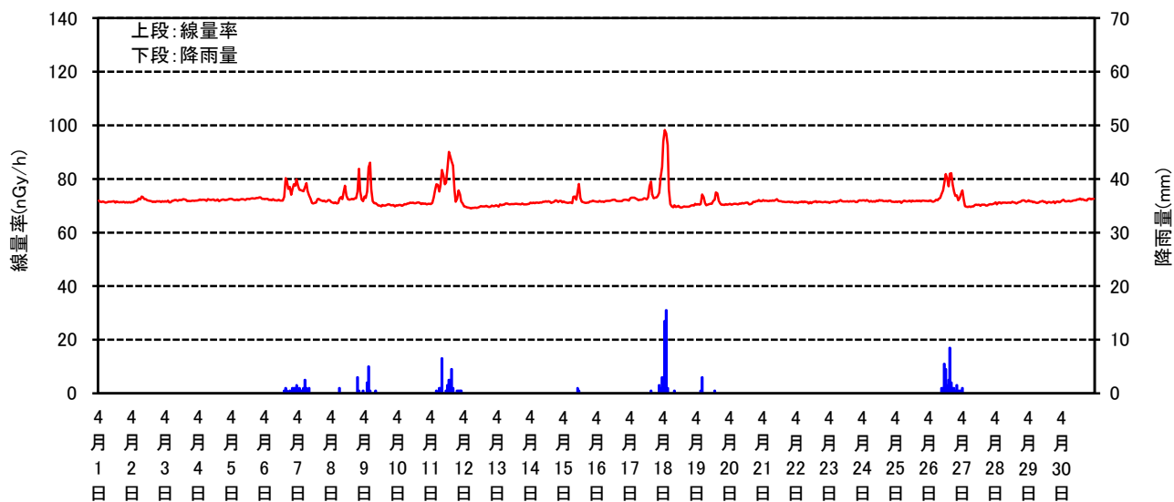
空間線量率と降雨量の測定結果(平成29年04月)
