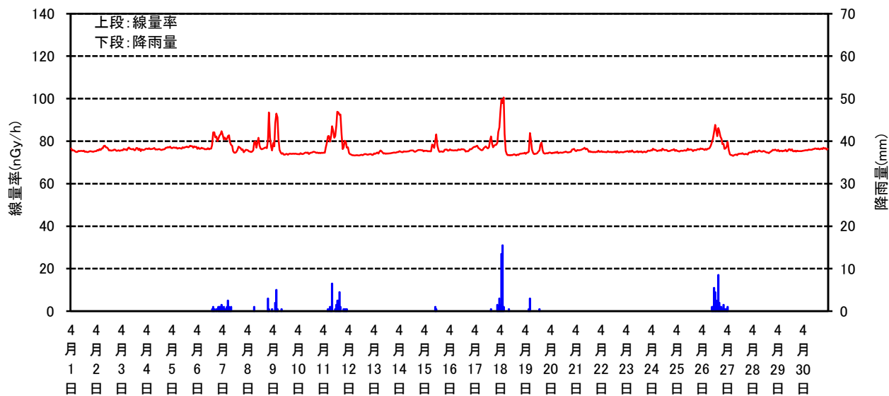
空間線量率と降雨量の測定結果(平成29年04月)
