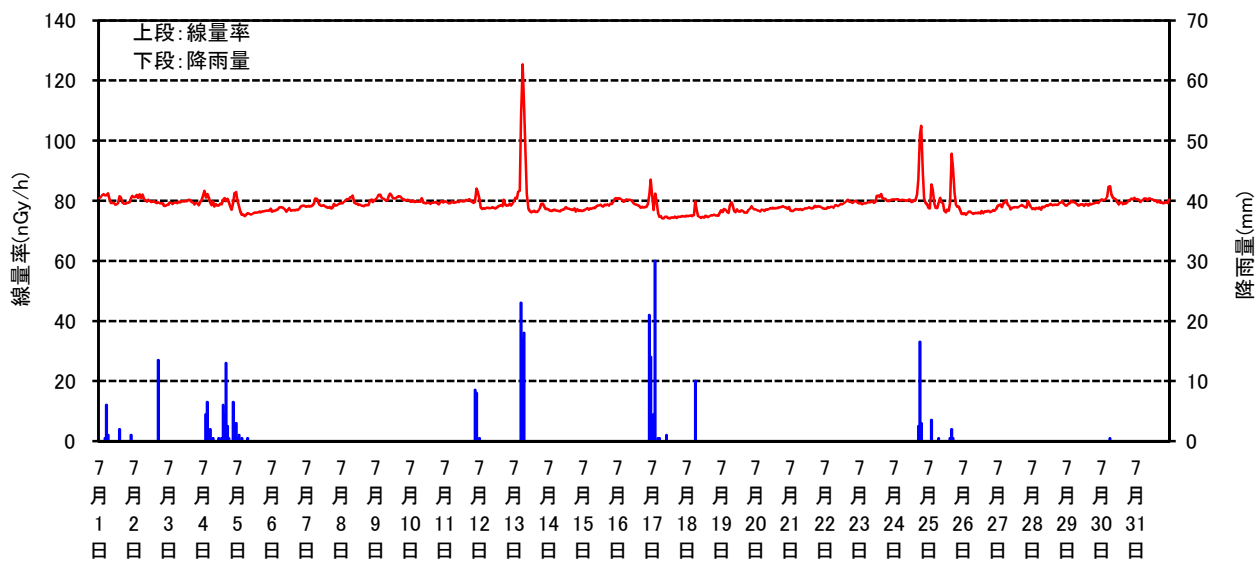
空間線量率と降雨量の測定結果(平成29年07月)
