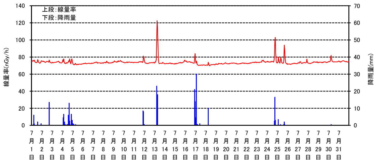
空間線量率と降雨量の測定結果(平成29年07月)
