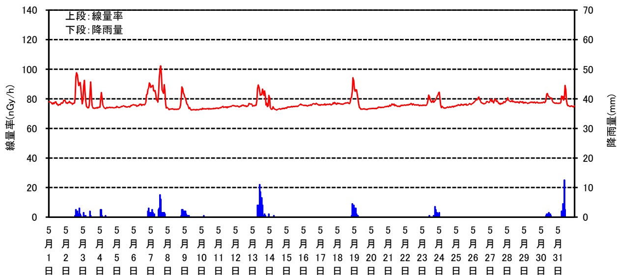
空間線量率と降雨量の測定結果(平成30年05月)
