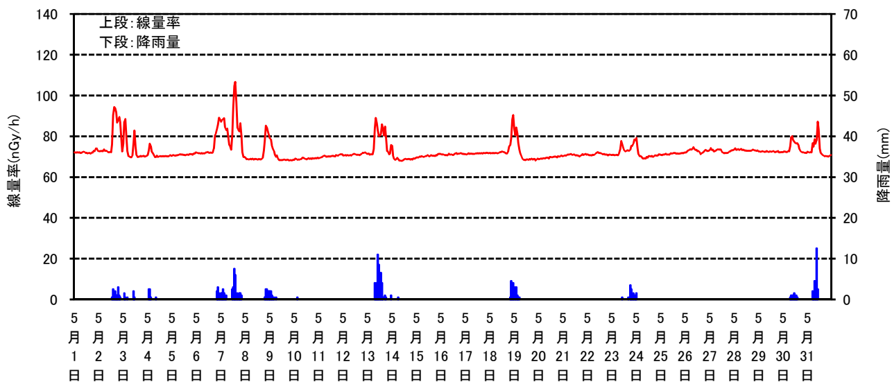
空間線量率と降雨量の測定結果(平成30年05月)
