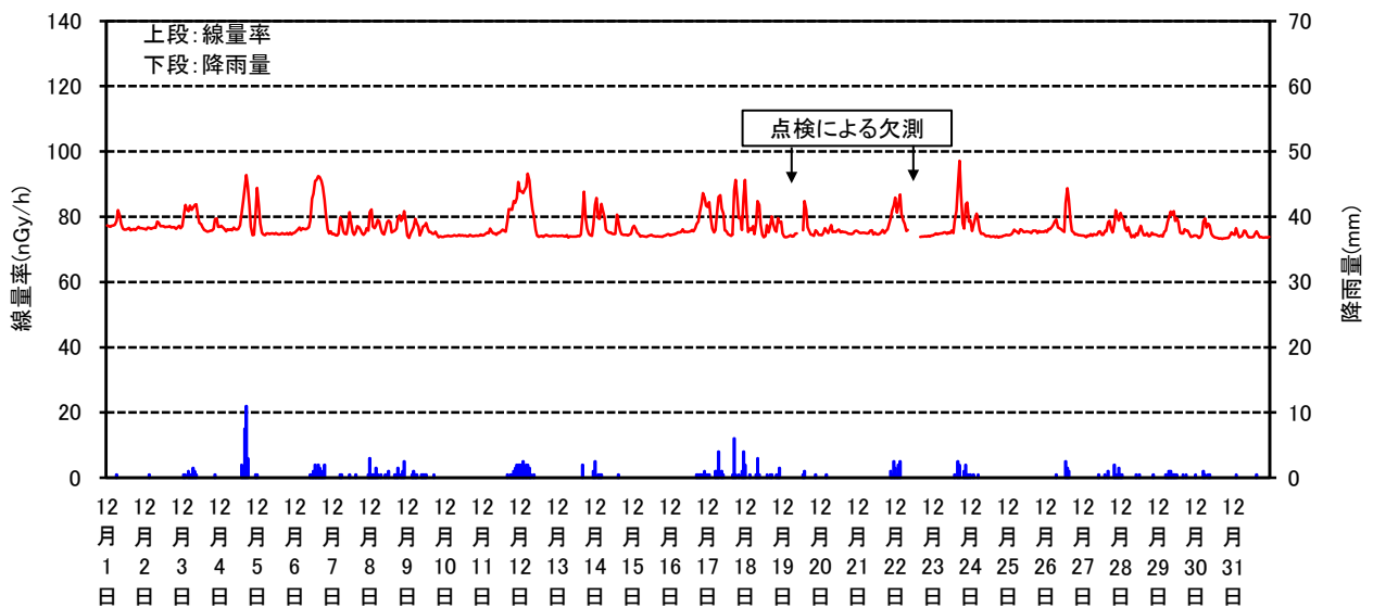
空間線量率と降雨量の測定結果(平成30年12月)
