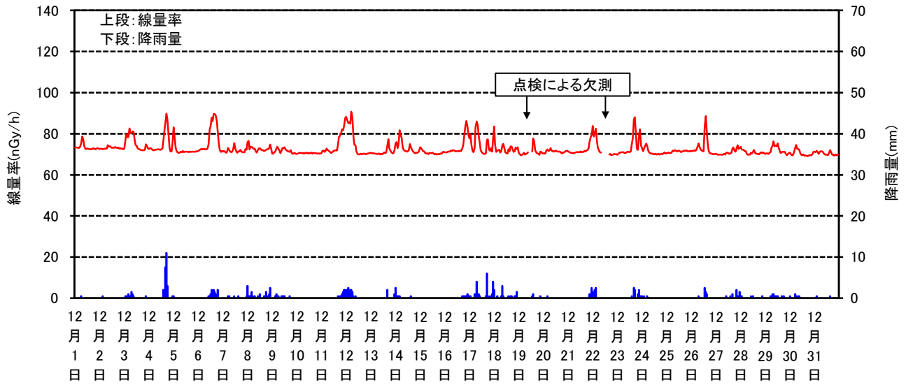
空間線量率と降雨量の測定結果(平成30年12月)
