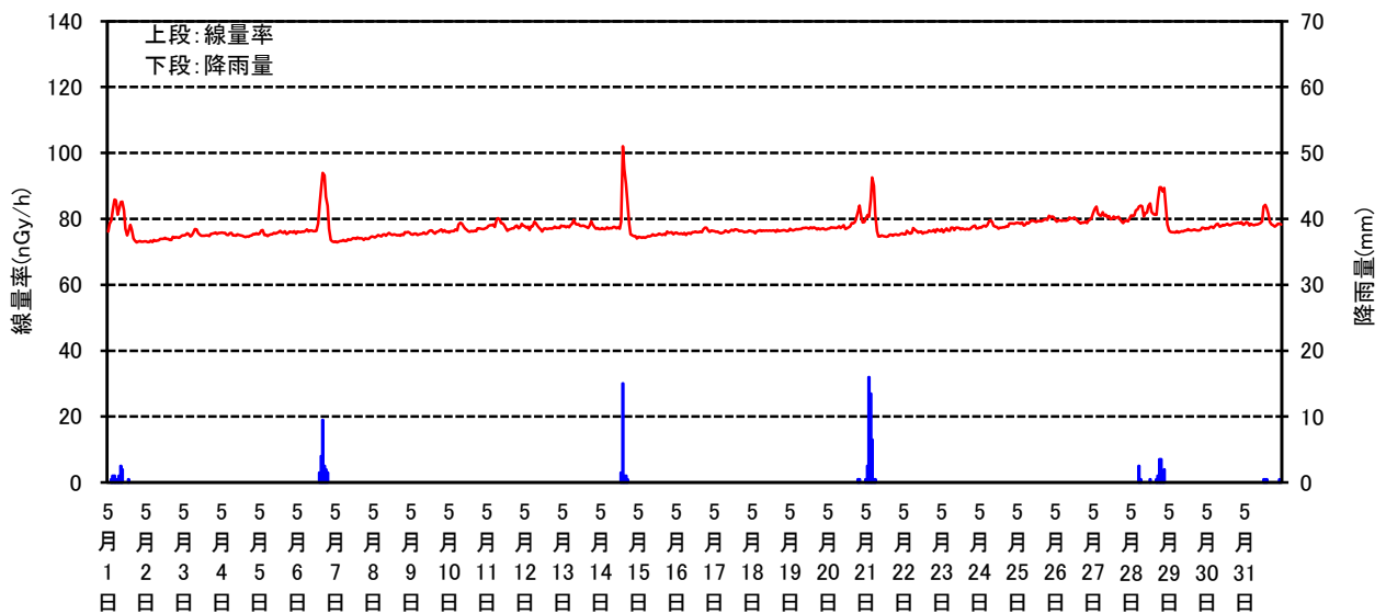
空間線量率と降雨量の測定結果(2019年05月)
