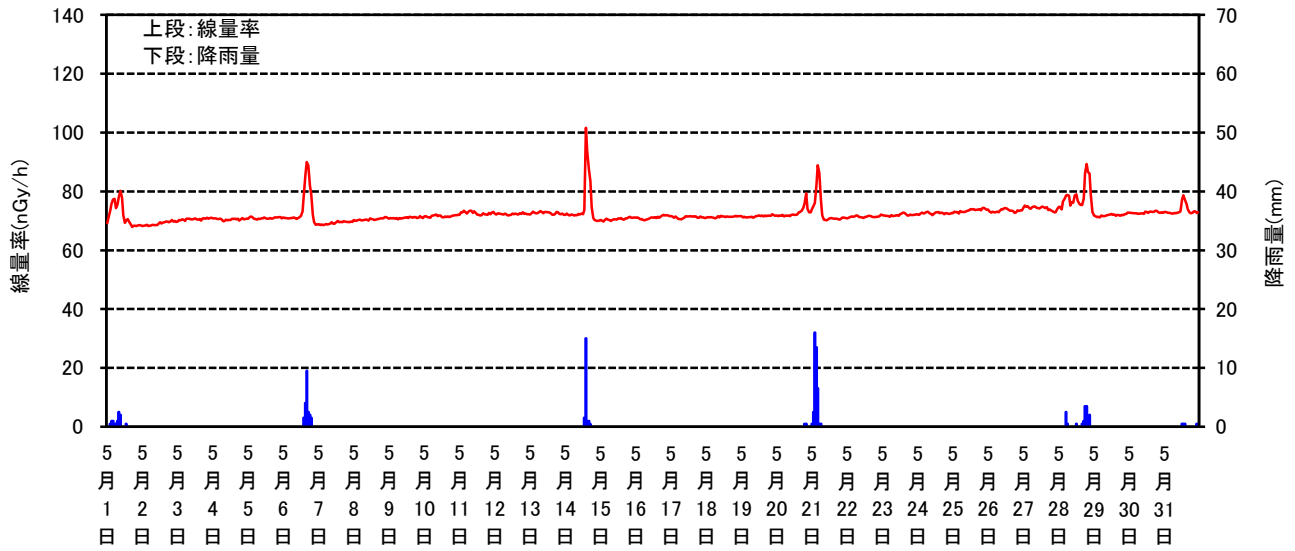
空間線量率と降雨量の測定結果(2019年05月)
