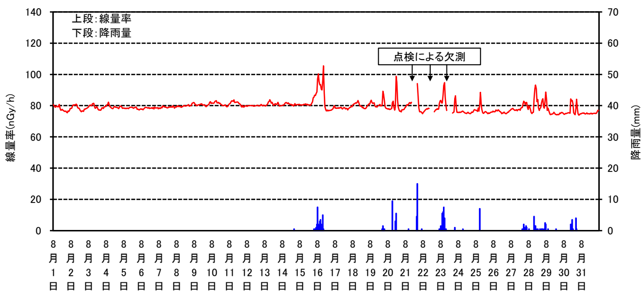
空間線量率と降雨量の測定結果(2019年08月)
