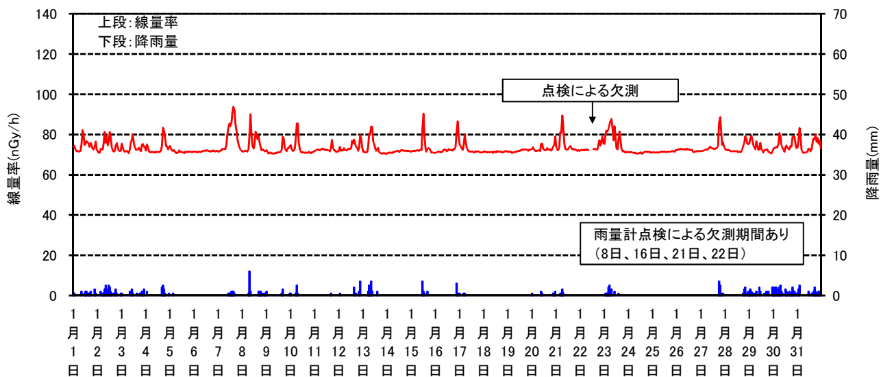
空間線量率と降雨量の測定結果(2020年01月)
