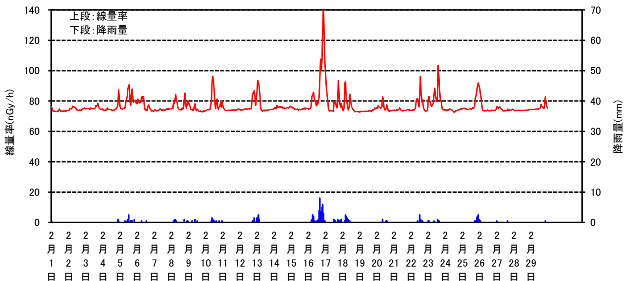
空間線量率と降雨量の測定結果(2020年02月)
