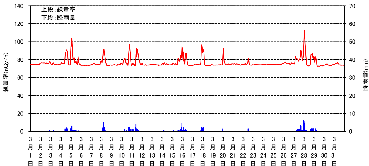
空間線量率と降雨量の測定結果(2020年03月)
