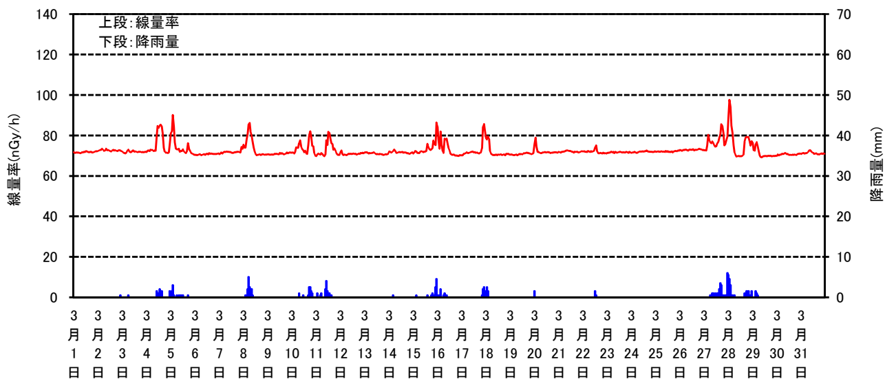
空間線量率と降雨量の測定結果(2020年03月)
