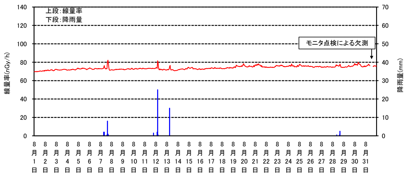
空間線量率と降雨量の測定結果(2020年08月)
