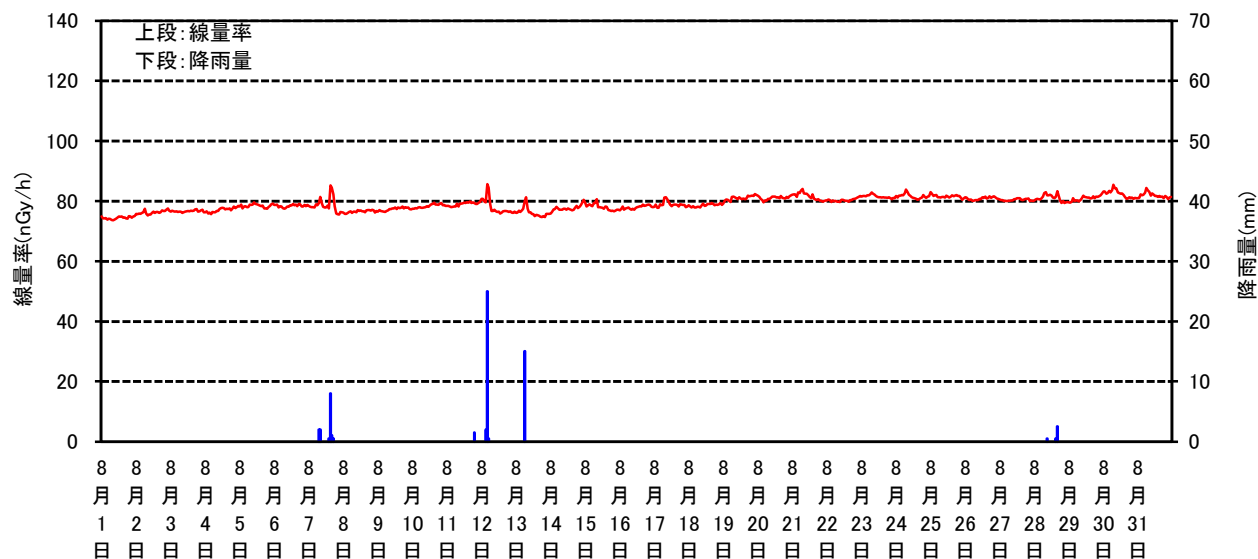
空間線量率と降雨量の測定結果(2020年08月)
