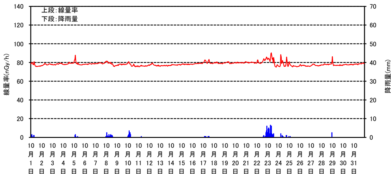
空間線量率と降雨量の測定結果(2020年10月)
