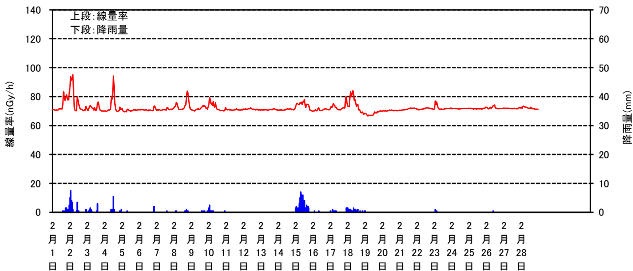
空間線量率と降雨量の測定結果(2021年02月)
