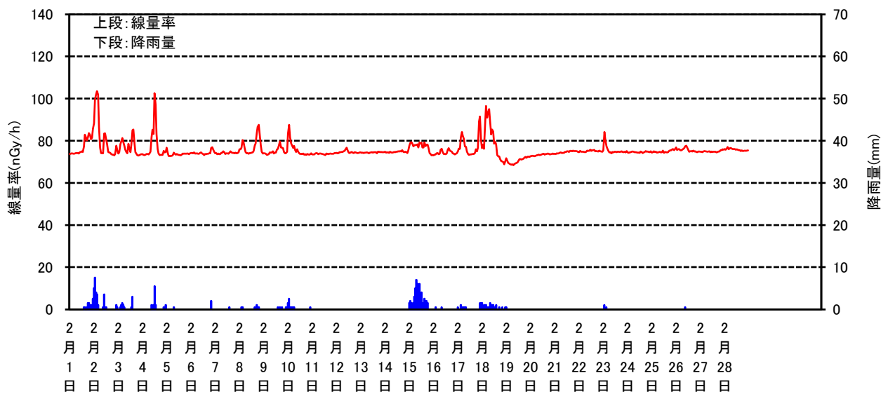
空間線量率と降雨量の測定結果(2021年02月)
