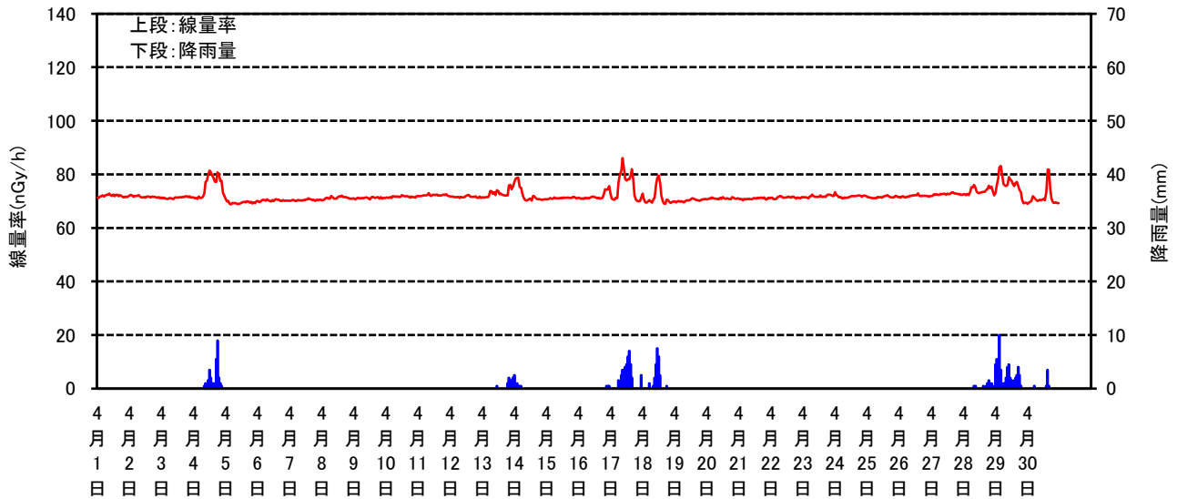
空間線量率と降雨量の測定結果(2021年04月)
