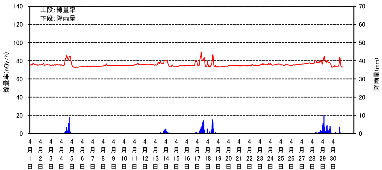
空間線量率と降雨量の測定結果(2021年04月)
