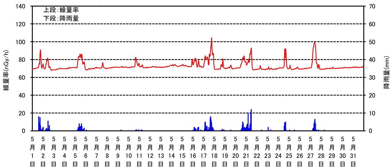
空間線量率と降雨量の測定結果(2021年05月)
