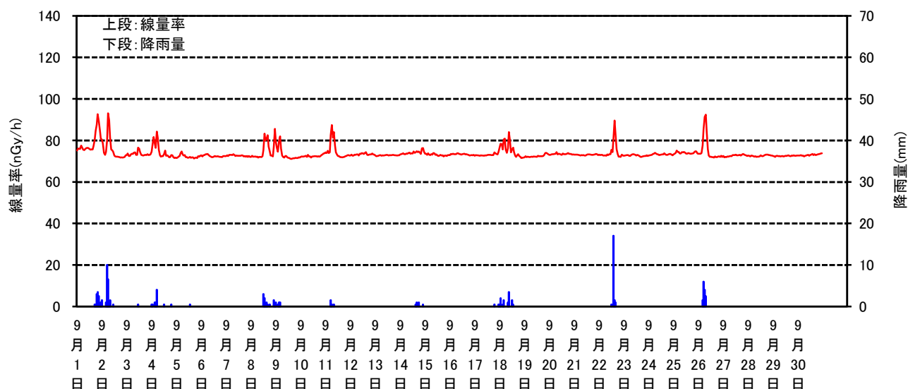
空間線量率と降雨量の測定結果(2021年09月)
