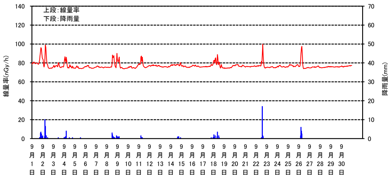
空間線量率と降雨量の測定結果(2021年09月)
