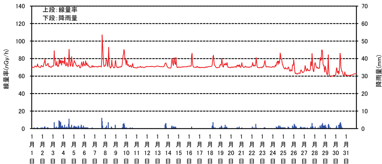
空間線量率と降雨量の測定結果(2023年01月)
