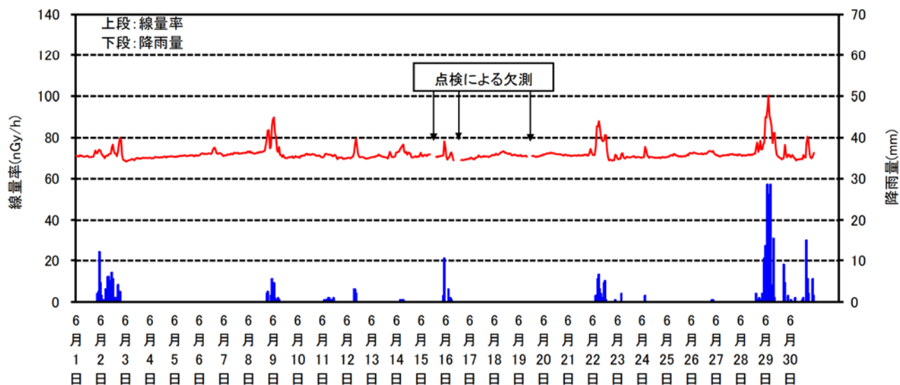
空間線量率と降雨量の測定結果(2023年6月)
