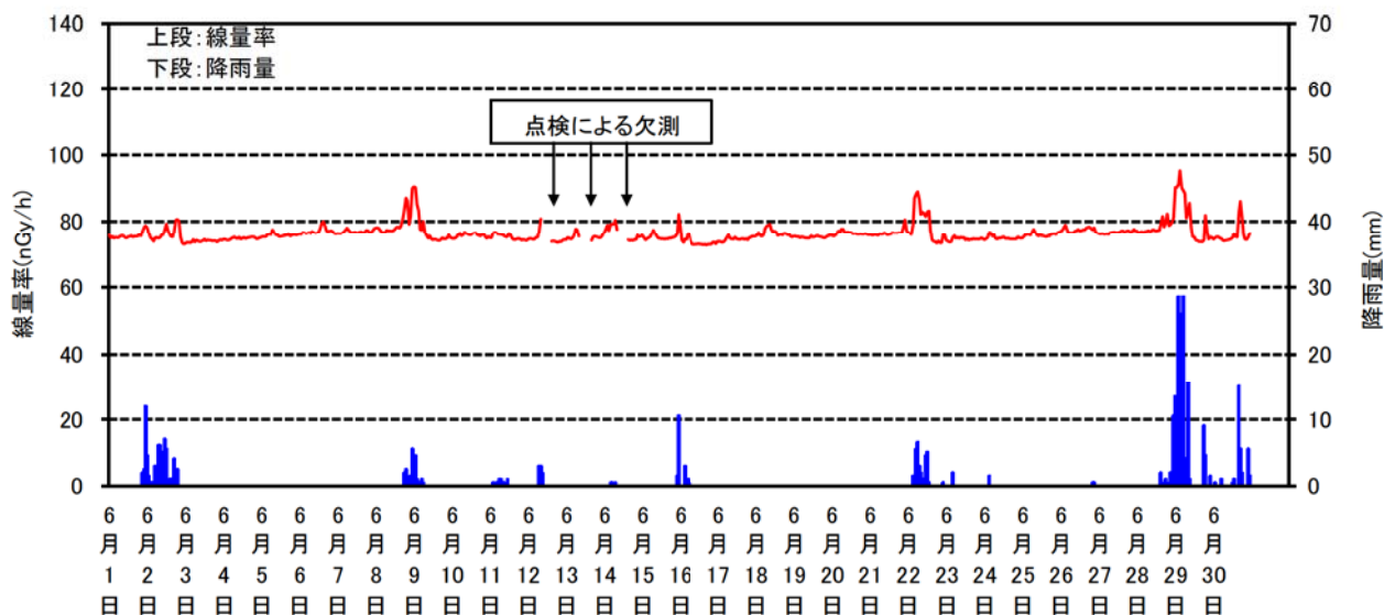
空間線量率と降雨量の測定結果(2023年6月)
