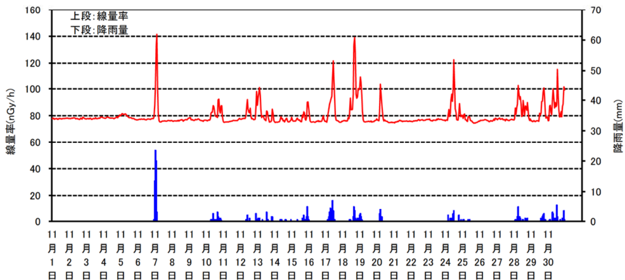
空間線量率と降雨量の測定結果(2023年11月)
