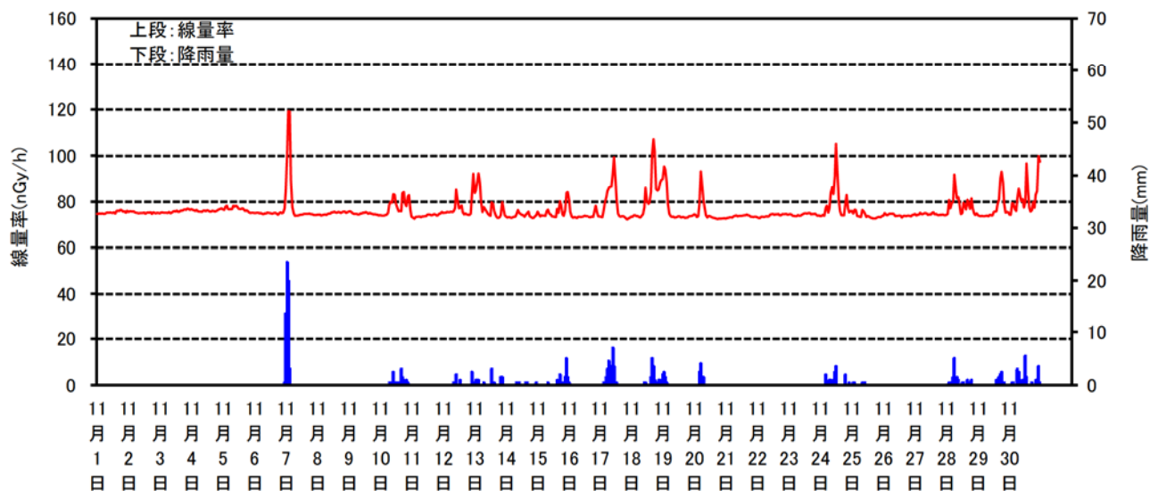
空間線量率と降雨量の測定結果(2023年11月)
