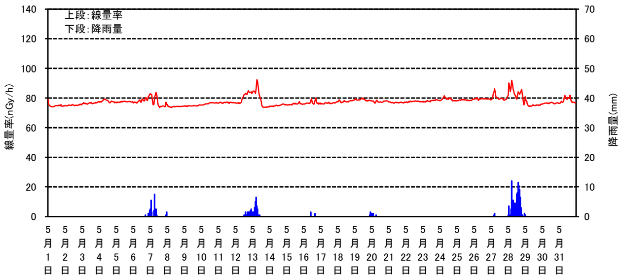
空間線量率と降雨量の測定結果(2024年5月)
