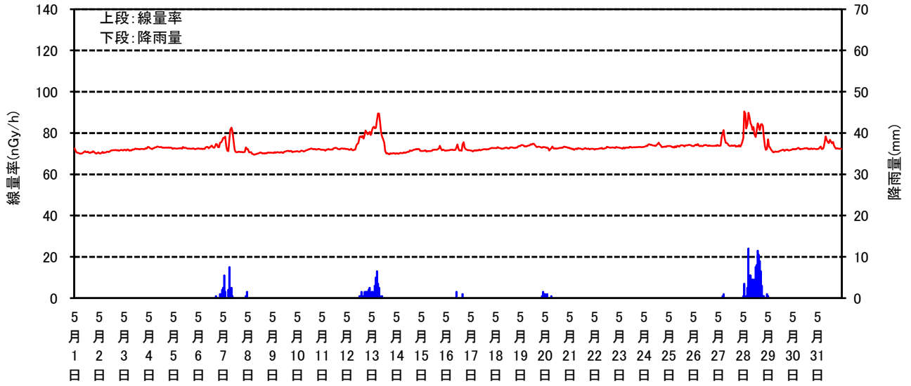
空間線量率と降雨量の測定結果(2024年5月)
