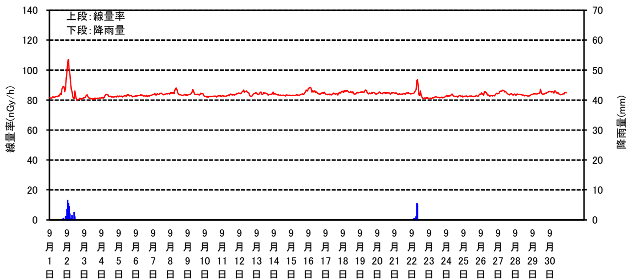
空間線量率と降雨量の測定結果(2024年9月)
