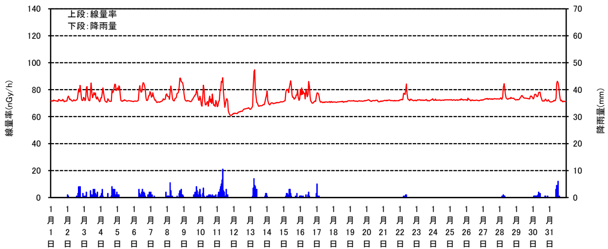
空間線量率と降雨量の測定結果(2025年1月)
