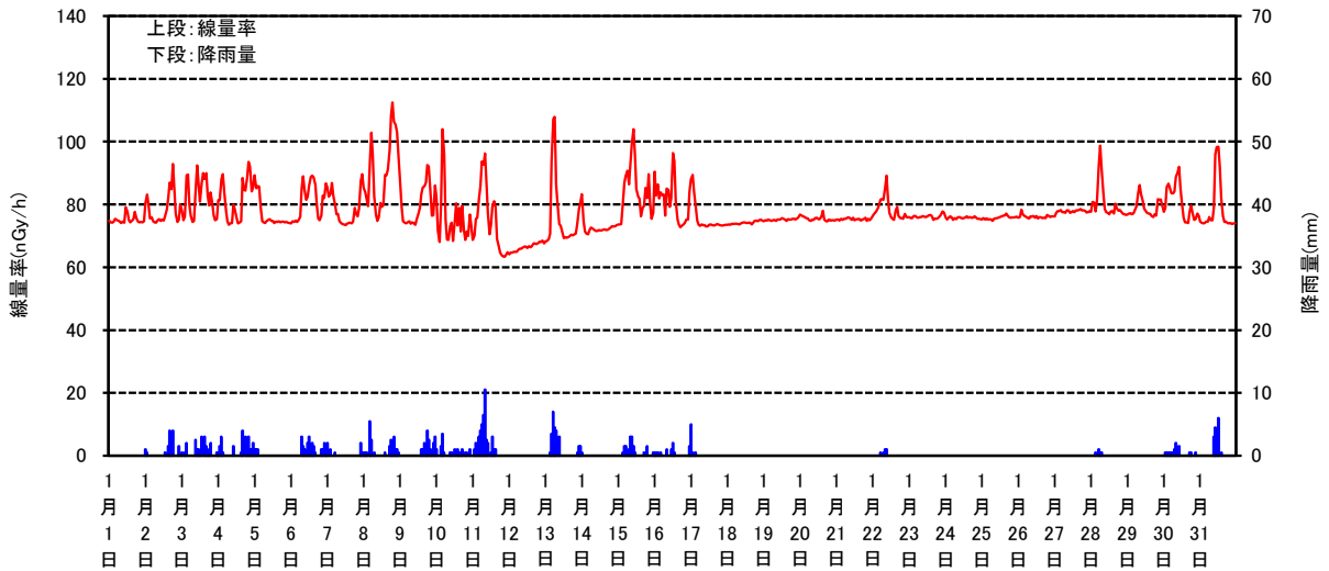
空間線量率と降雨量の測定結果(2025年1月)
