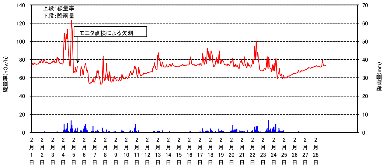
空間線量率と降雨量の測定結果(2025年2月)
