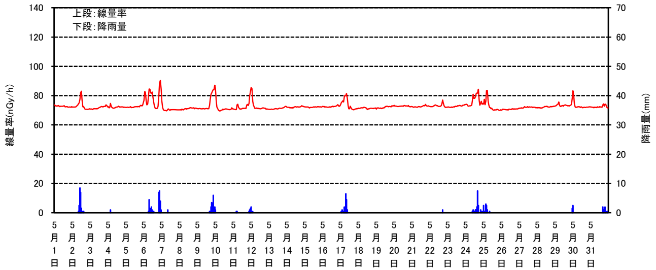
空間線量率と降雨量の測定結果(2025年5月)
