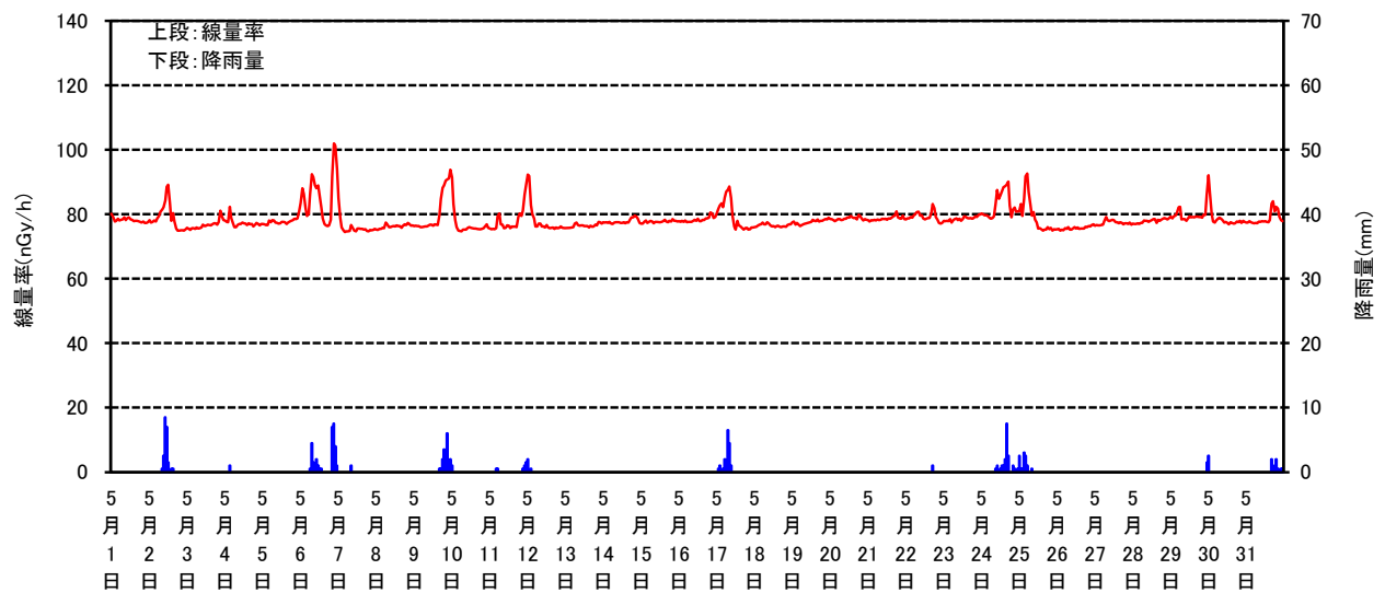
空間線量率と降雨量の測定結果(2025年5月)
