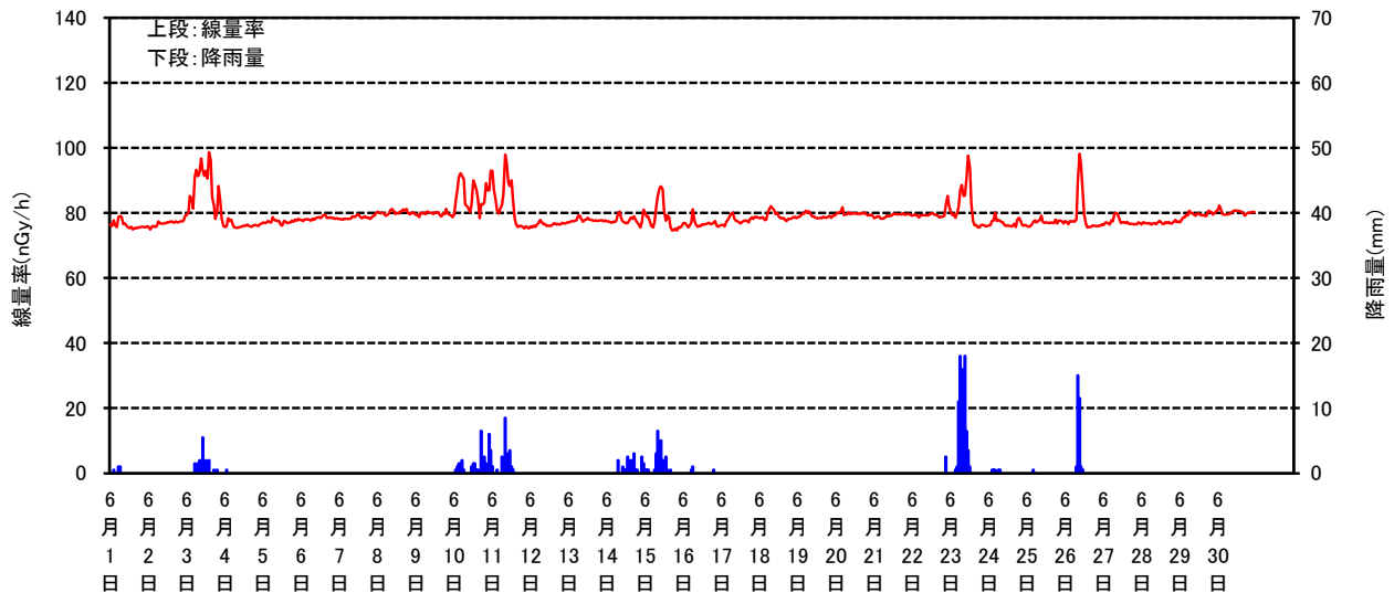
空間線量率と降雨量の測定結果(2025年6月)
