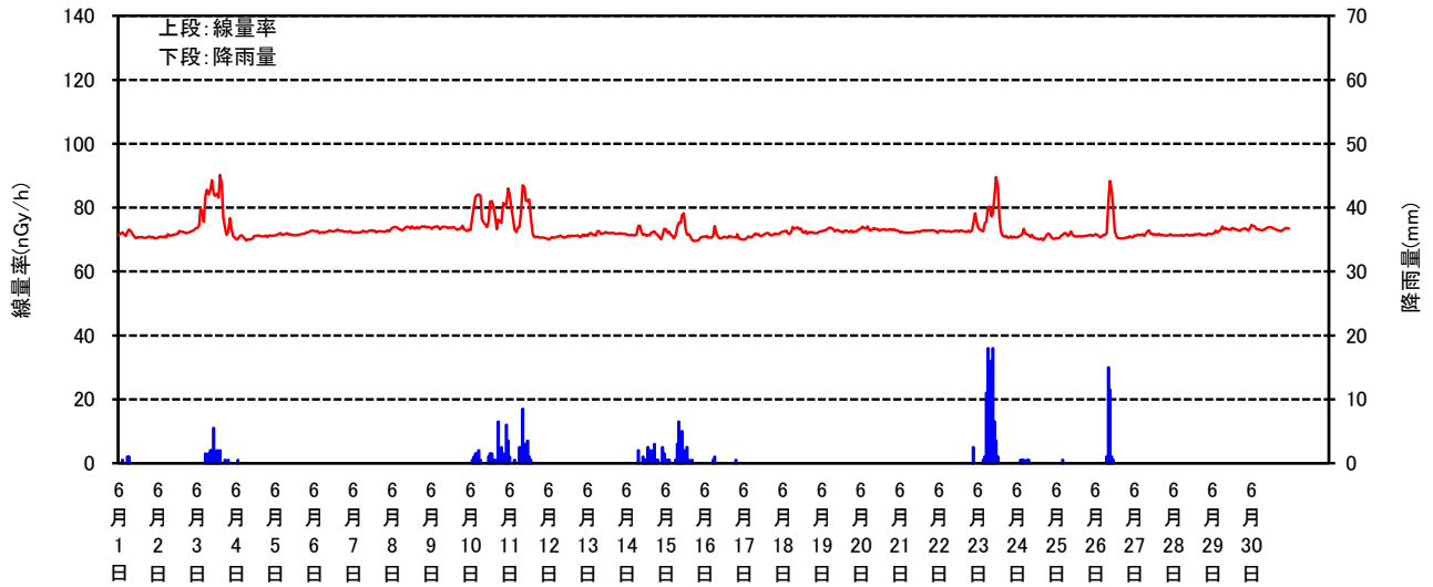
空間線量率と降雨量の測定結果(2025年6月)
