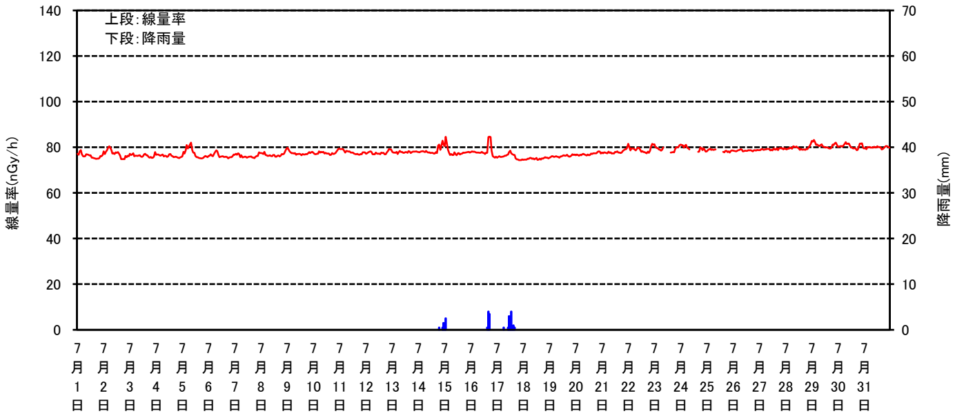
空間線量率と降雨量の測定結果(2025年7月)
