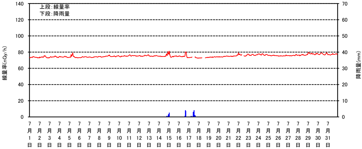
空間線量率と降雨量の測定結果(2025年7月)
