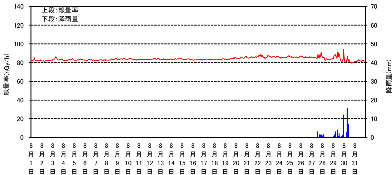
空間線量率と降雨量の測定結果(2026年8月)
