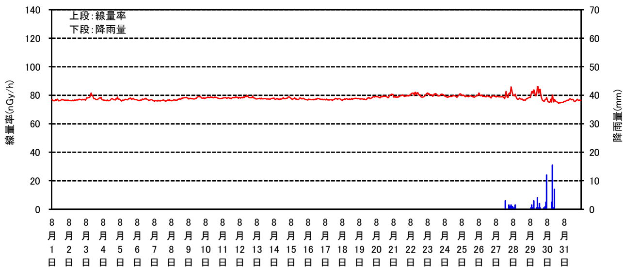
空間線量率と降雨量の測定結果(2026年8月)
