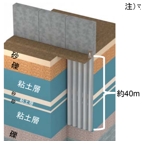
摩擦杭(北側)
