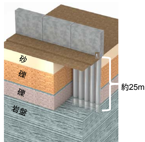
支持杭(南側)
