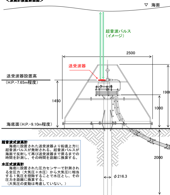
<波高計設置断面図>
