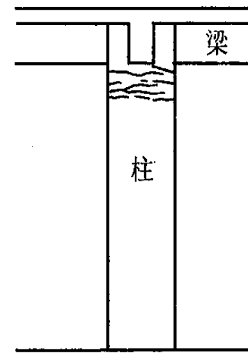
【柱に生じる地震時ひび割れ発生例】
