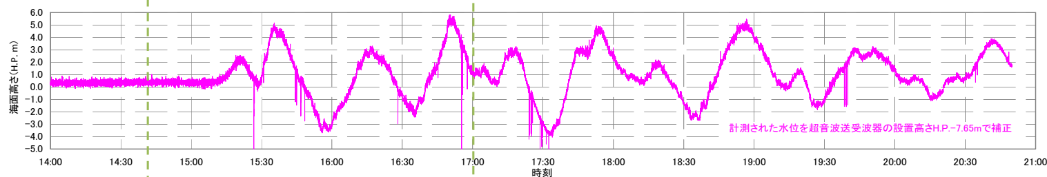
水位変動(水圧式波高計より)
