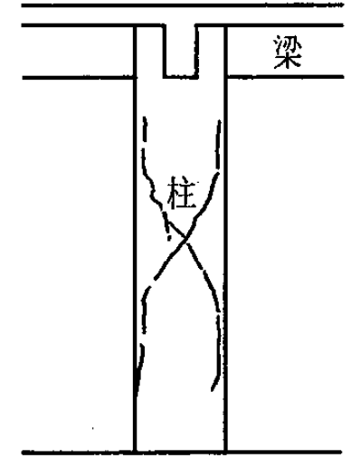
【柱に生じる地震時ひび割れ発生例】
