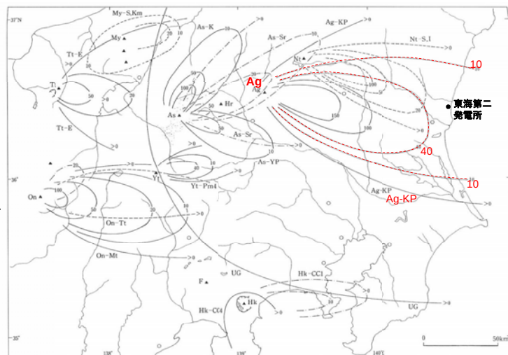
図 3.3-2 中部・関東地方の後期更新世主要テフラの等層厚線図(その1) Nt-S 男体七郎山 (1) Nt-I 男体今市 (1) UG 立川ローム上部ガラス質 (2) As-K 浅間草津 (pH の分布も示す) (3) As-YP 浅間御嶽 (pH の分布も示す) (3) As-Sr 浅間白糸 (4) Yt-Pm4 ハッ岳 (5) Ag-KP 赤城鹿沼 (6) My-S-Km 砂島山・兼良 (7) Hk-CC4 箱根三島 (8) Hk-CC1 箱根中央火口丘 (9) Tt-E 立山 (10) On-Mt 御岳三郎 (11) On-Tt 御岳三郎 (11) Tt: 立山, My: 砂島, As: 浅間, Hr: 榛名, Nt: 日光男体, On: 御岳, Yt: ハッ岳, F: 富士, Hk: 箱根, [1] 関東ローム研究グループ (1985), [2] 鈴木正幸 (1991), [3] 中沢ほか (1994), [4] Kawachi et al. (1987), [5] 中谷 (1970), [6] 鈴木 (1980), [7] 早津・新井 (1980), [8] 町田 (1971), [9] 町田 (1982), [10] 竹本ほか (1987)
