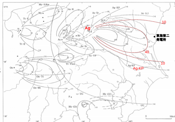
図 3.3-2 中部・関東地方の後期更新世主要テフラの等層厚線図(その1) Nt-S 男体七郎山 (1)(2)(3)(4) Nt-I 男体今市 (1)(2)(3)(4) UG 立川ローム上部ガラス質 (2)(3) As-K 浅間草津 (pH の分布も示す) (3) As-YP 浅間御嶽 (pH の分布も示す) (3) As-Sr 浅間白糸 (3) Yt-Pm4 ハッ岳 (4)(5) Ag-KP 赤城鹿沼 (1)(2) My-S-Km 砂島山・兼良 (2)(3) Hk-CC4 箱根三島 (2) Hk-CC1 箱根中央火口丘 (1)(2) Yt-E 立山 (2)(3)(4) On-Mt 御岳三郎 (2)(3) On-Tt 御岳三郎 (2)(3) Tt-I 立山 My-砂島 As-浅間 Hr-鎌名 Nt-日光男体 On-御岳 Yt-ハッ岳 F-富士 Hk-箱根 (1) 関東ローム研究グループ (1985), (2) 鈴木正幸 (1991), (3) 中沢ほか (1994), (4) Kawachi et al. (1987), (5) 中谷 (1970), (6) 鈴木 (1980), (7) 早津・新井 (1980), (8) 町田 (1971), (9) 町田 (1982), (10) 竹本ほか (1987)
