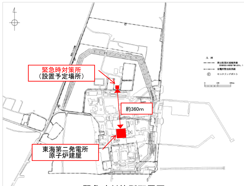
緊急時対策所配置図
