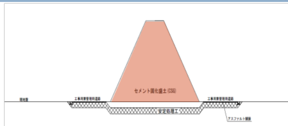
敷地全体 断面イメージ図
