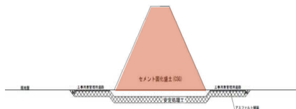
＜防潮堤の概要＞
