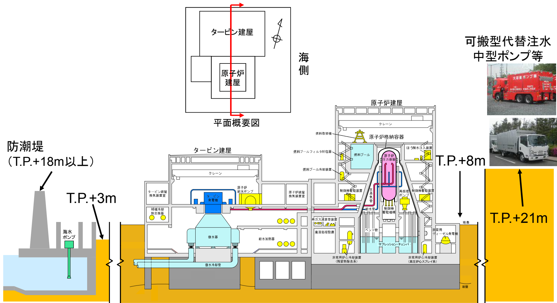
建屋断面は南南東—北北西方向
