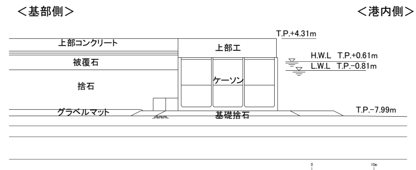
ケーソン堤断面図(②断面)
