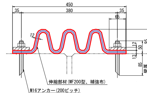
ジョイント例
