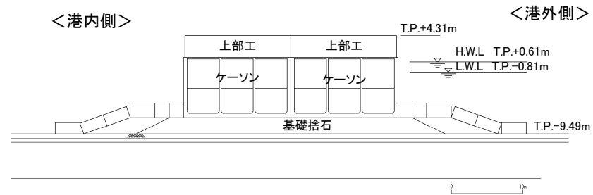
ケーソン堤断面図(①断面)
