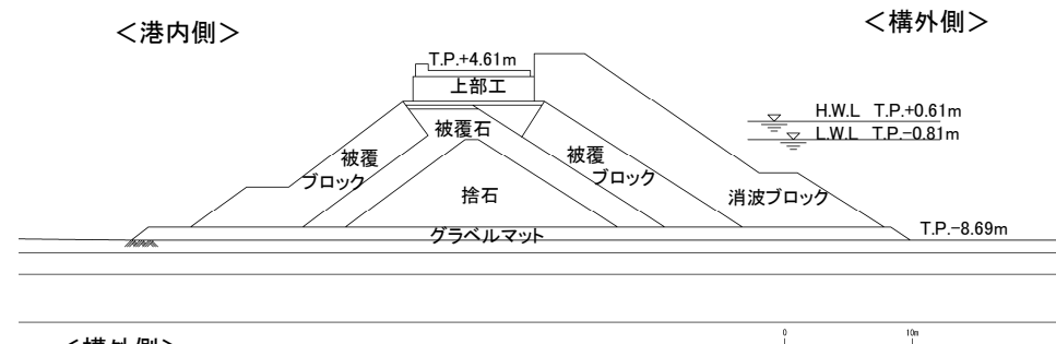
傾斜堤断面図(③断面)
