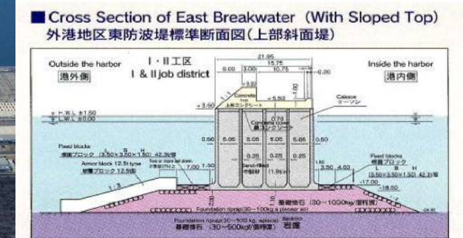
東防波堤標準構造
