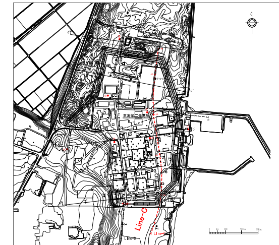
地質層序表
