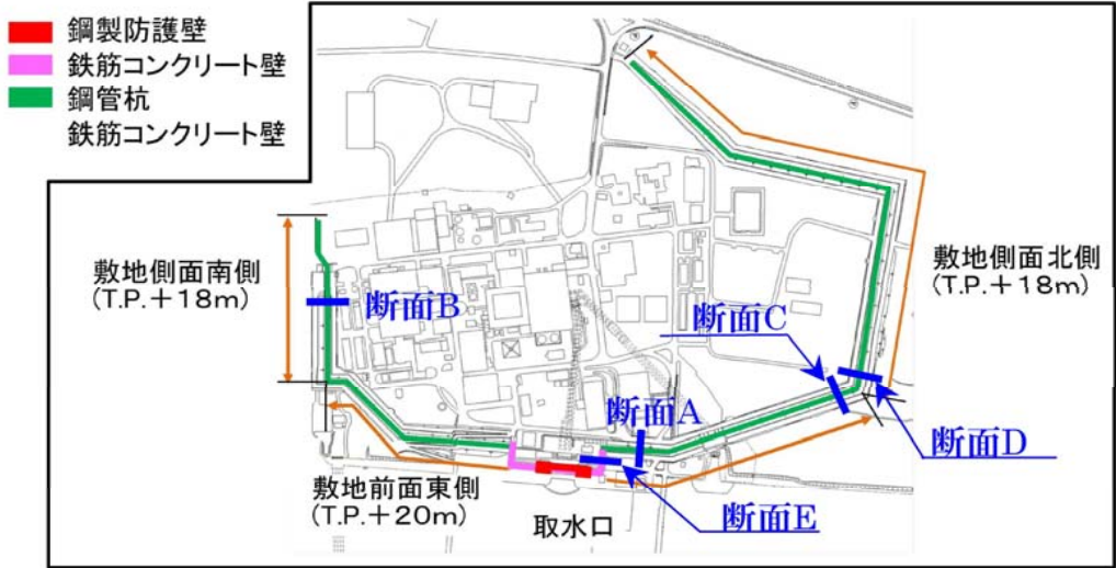
断面位置図
