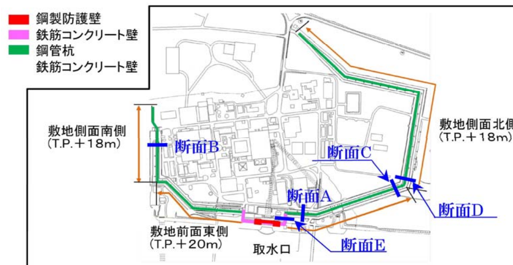
断面位置図
