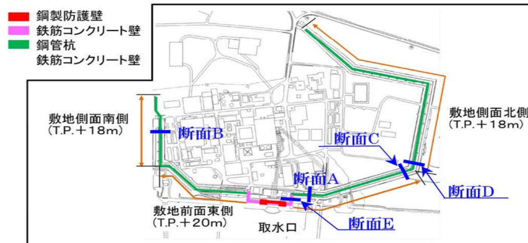
断面位置図
