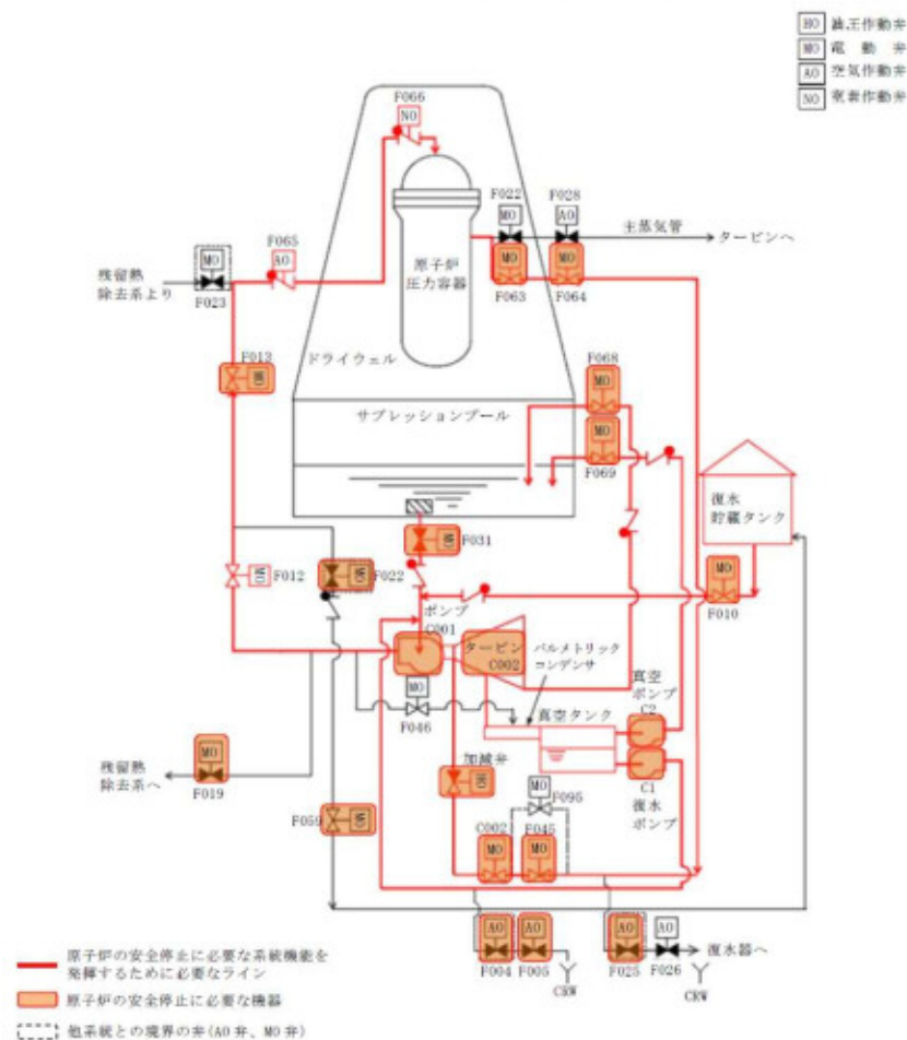
第 4 圖 原子炉隔離時冷却系
