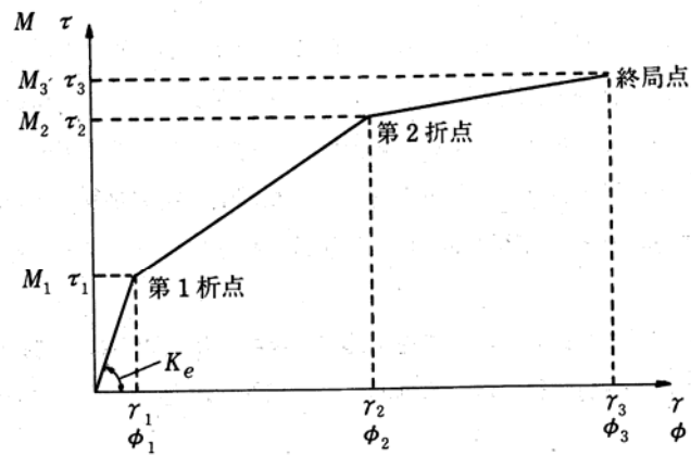
図4-1 トリリニヤー・スケルトンカーブ
