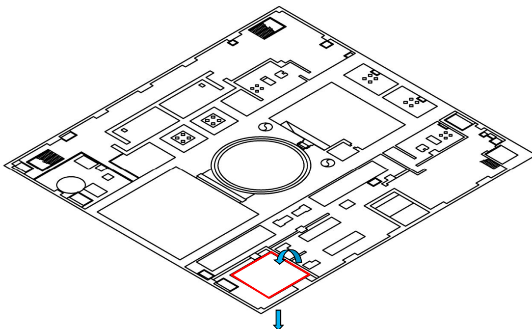
第 2 図 機器ハッチ部
