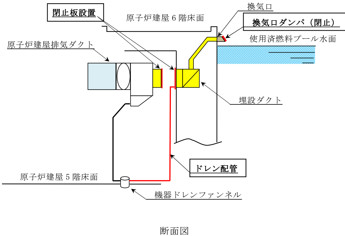
第 5 図 閉止板設置箇所
