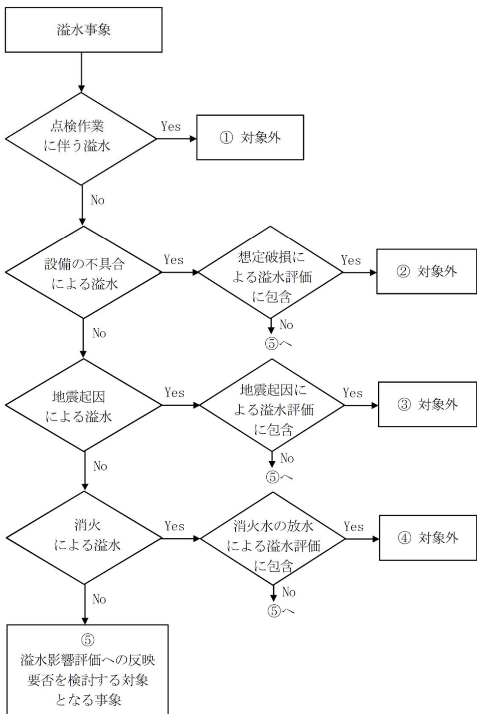
第 1 図 内部洪水影響評価への反映要否判断フロー
