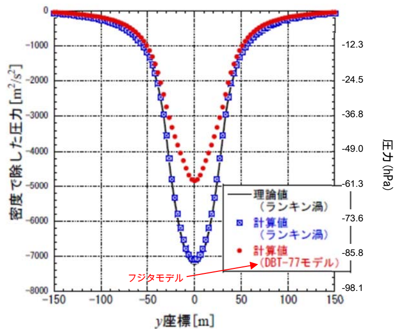
竜巻中心軸断面での密度で除した圧力分布 (最大接線風速 85m/s の場合)
