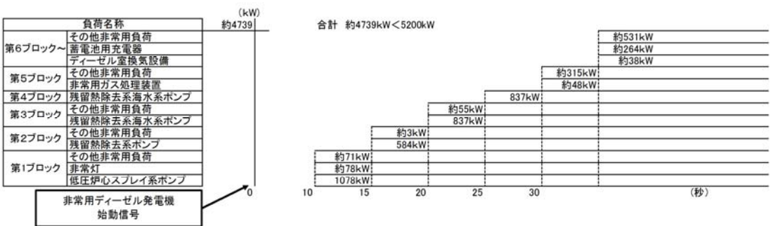
第 2.3.1.2-1 図 非常用ディーゼル発電機（2C）の負荷の始動順位 (外部電源喪失及び原子炉冷却材喪失時)
