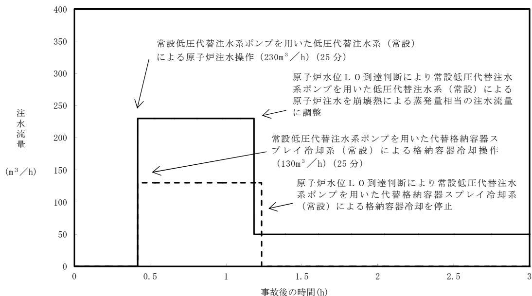
第 3. 1. 3-7 図 注水流量の推移 (短期挙動)
