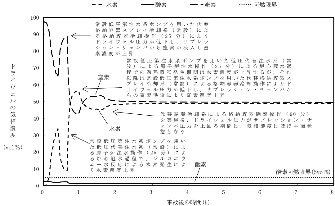
第 3.4-9 図 ドライウエルの気相濃度の推移（ドライ条件） （短期挙動）
