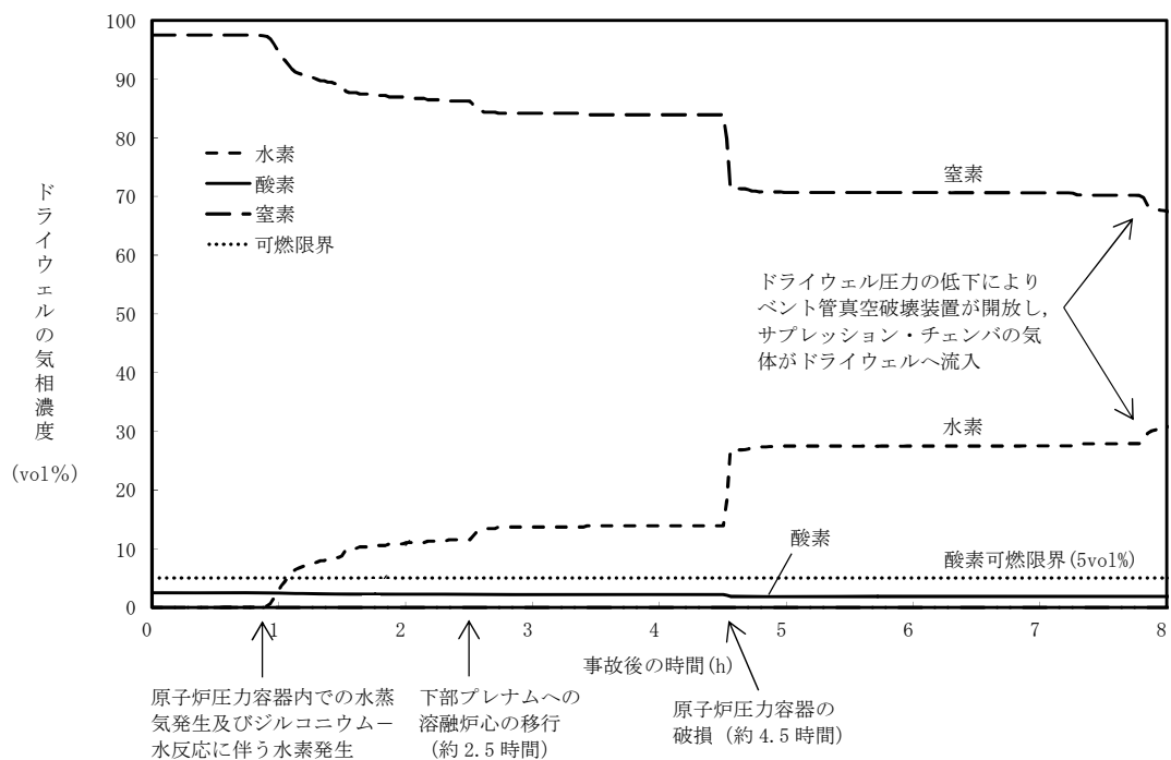
第 3.2-24 図 ドライウエルの気相濃度の推移 (ドライ条件) (～8 時間)
