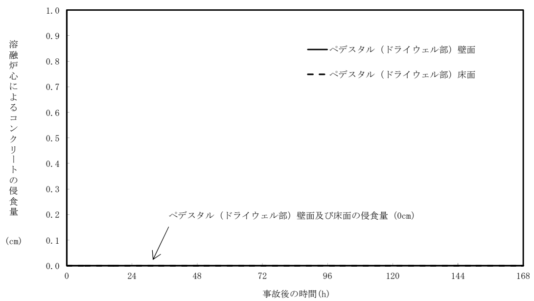
第 3.2-17 図 ペデスタル (ドライウェル部) の 壁面及び床面のコンクリート侵食量の推移
