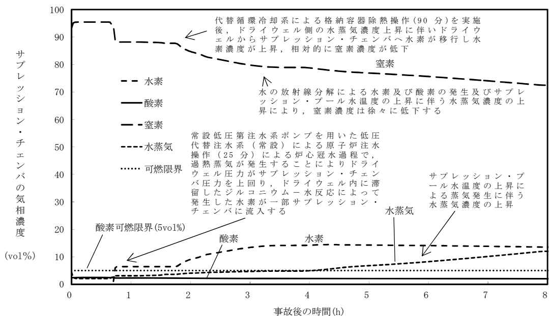
第 3.4-6 図 サプレッション・チェンバの気相濃度の推移 （ウェット条件）（短期挙動）
