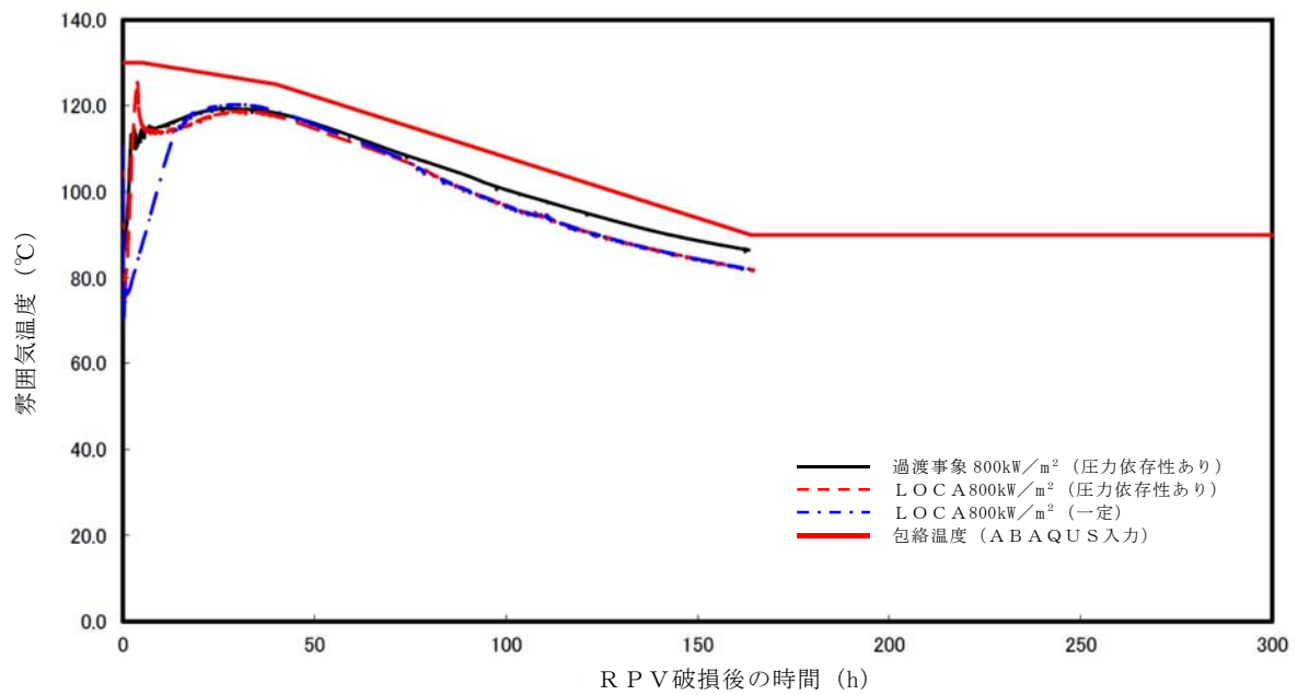
第 5 図 サプレッション・チェンバ蒸汽温度条件
