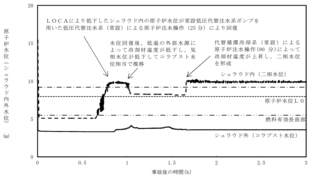
第 3. 1. 2-6 図 原子炉水位（シユラウド内外水位）の推移（短期挙動）
