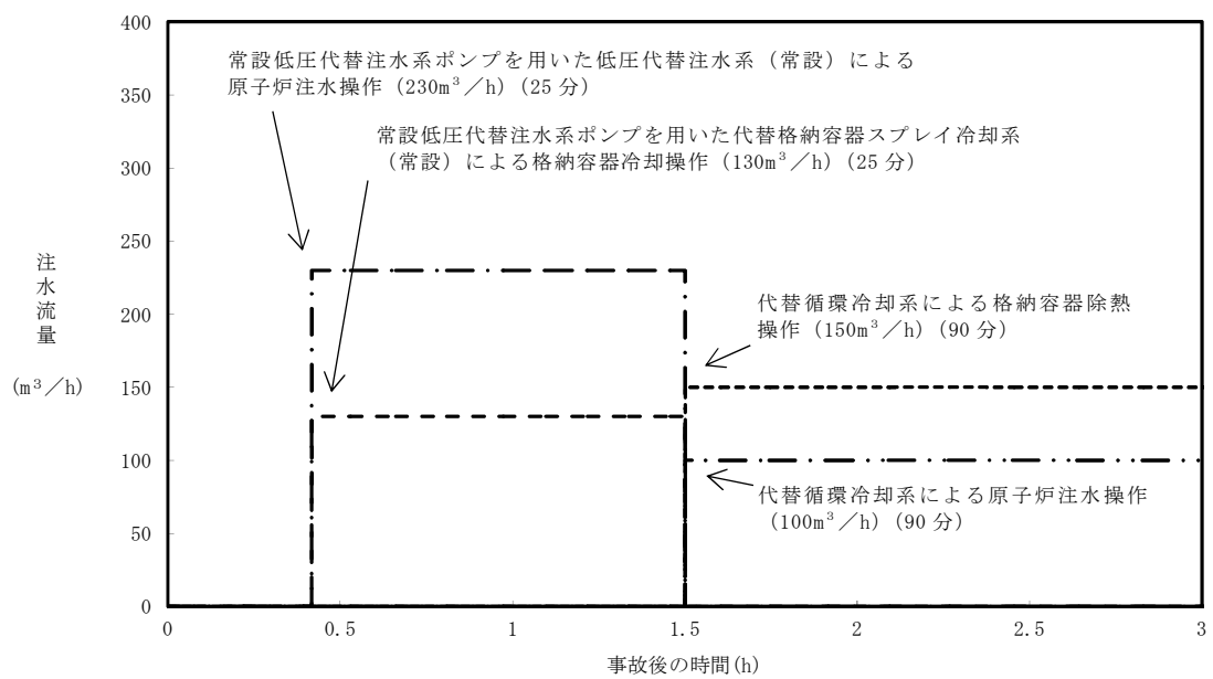
第 3. 1. 2-7 図 注水流量の推移（短期挙動）
