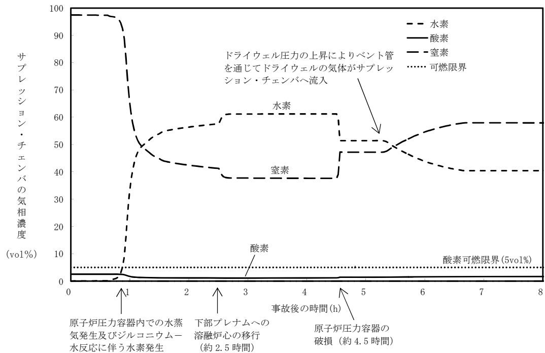
第 3.2-25 図 サブプレッション・チェンバの気相濃度の推移 (ドライ条件) (～8 時間)
