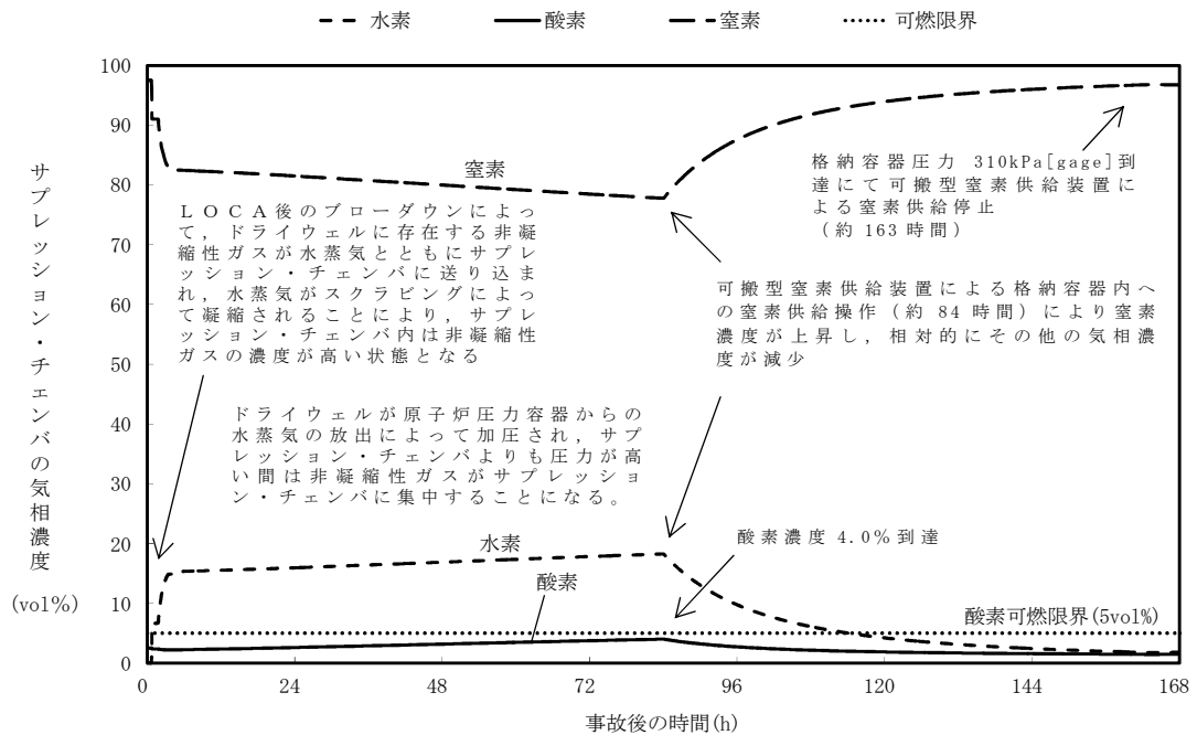
第 3.4-8 図 サブプレッション・チェンバの気相濃度の推移 (ドライ条件)
