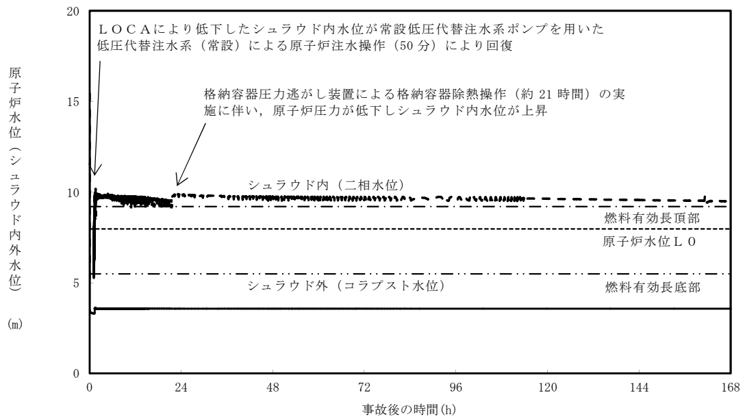
第 3.1.3-16 図 操作開始時間 25 分遅れのケースにおける原子炉水位 (シュラウド内外水位) の推移
