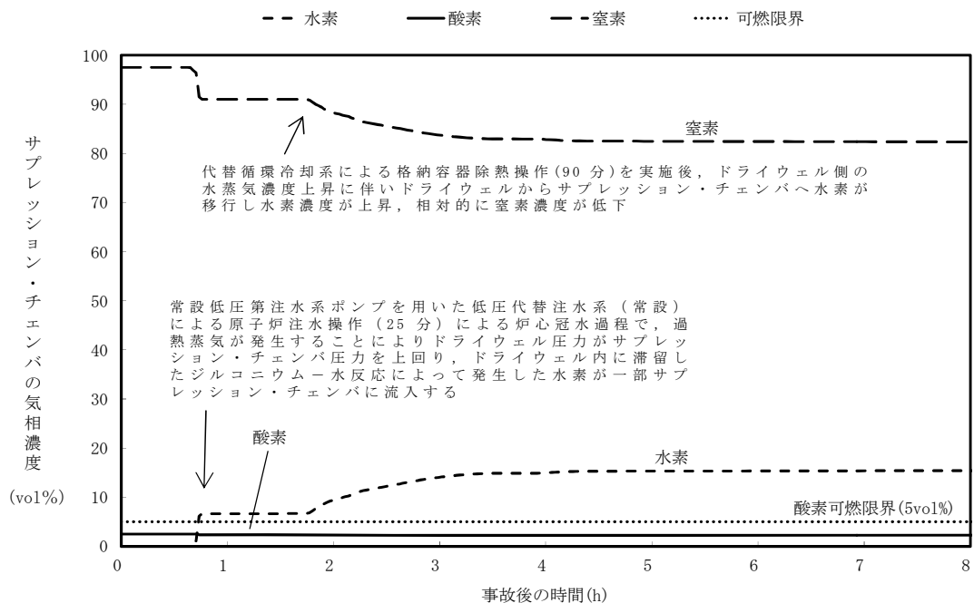
第 3.4-10 図 サプレッション・チェンバの気相濃度の推移 （ドライ条件）（短期挙動）
