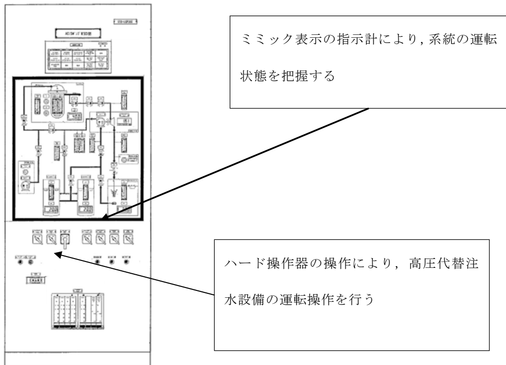
第 3 図 高圧代替注水系制御盤（イメージ図）
