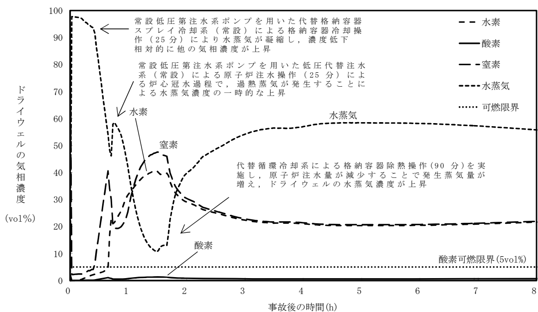
第 3.4-5 図 ドライウエルの気相濃度の推移（ウェット条件） （短期挙動）
