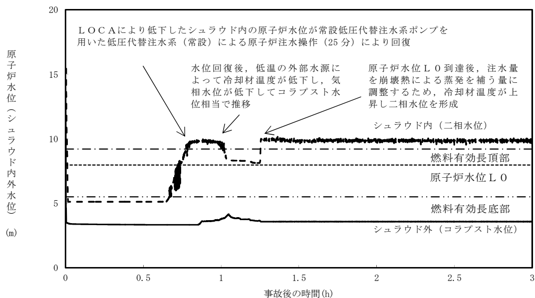
第 3. 1. 3-6 図 原子炉水位 (シュラウド内外水位) の推移 (短期挙動)
