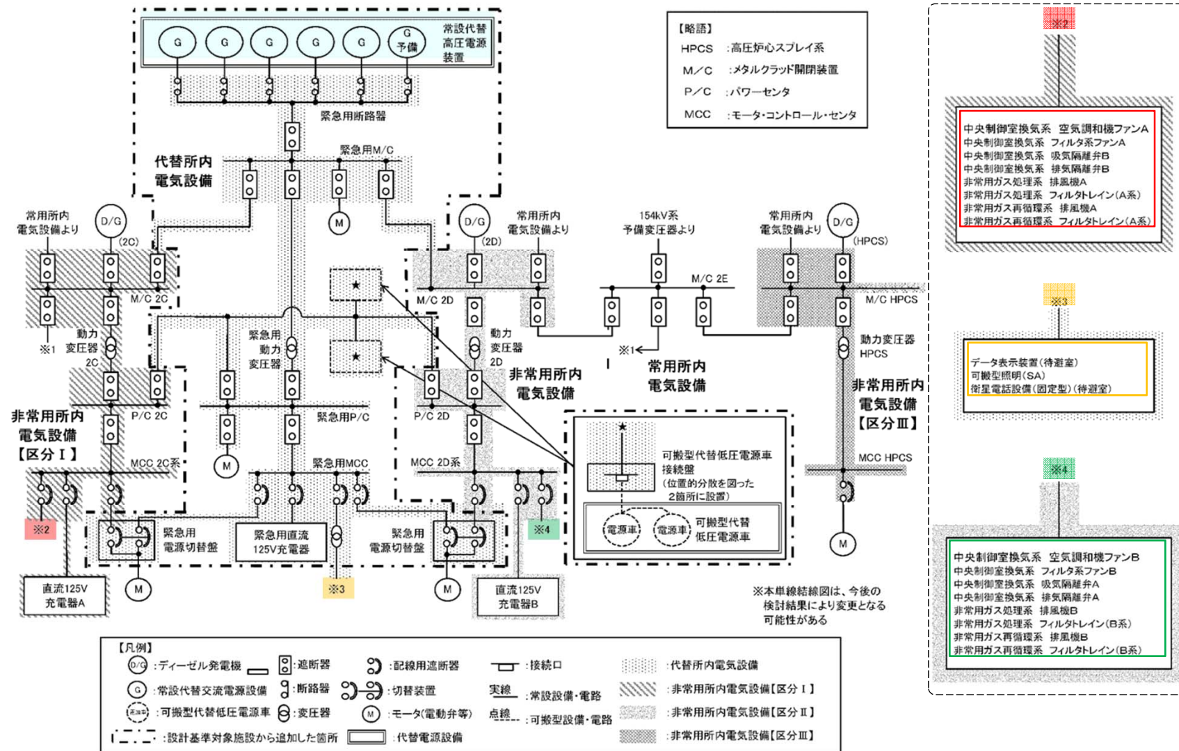
単線結線図
