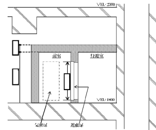
(A-A断面図)
