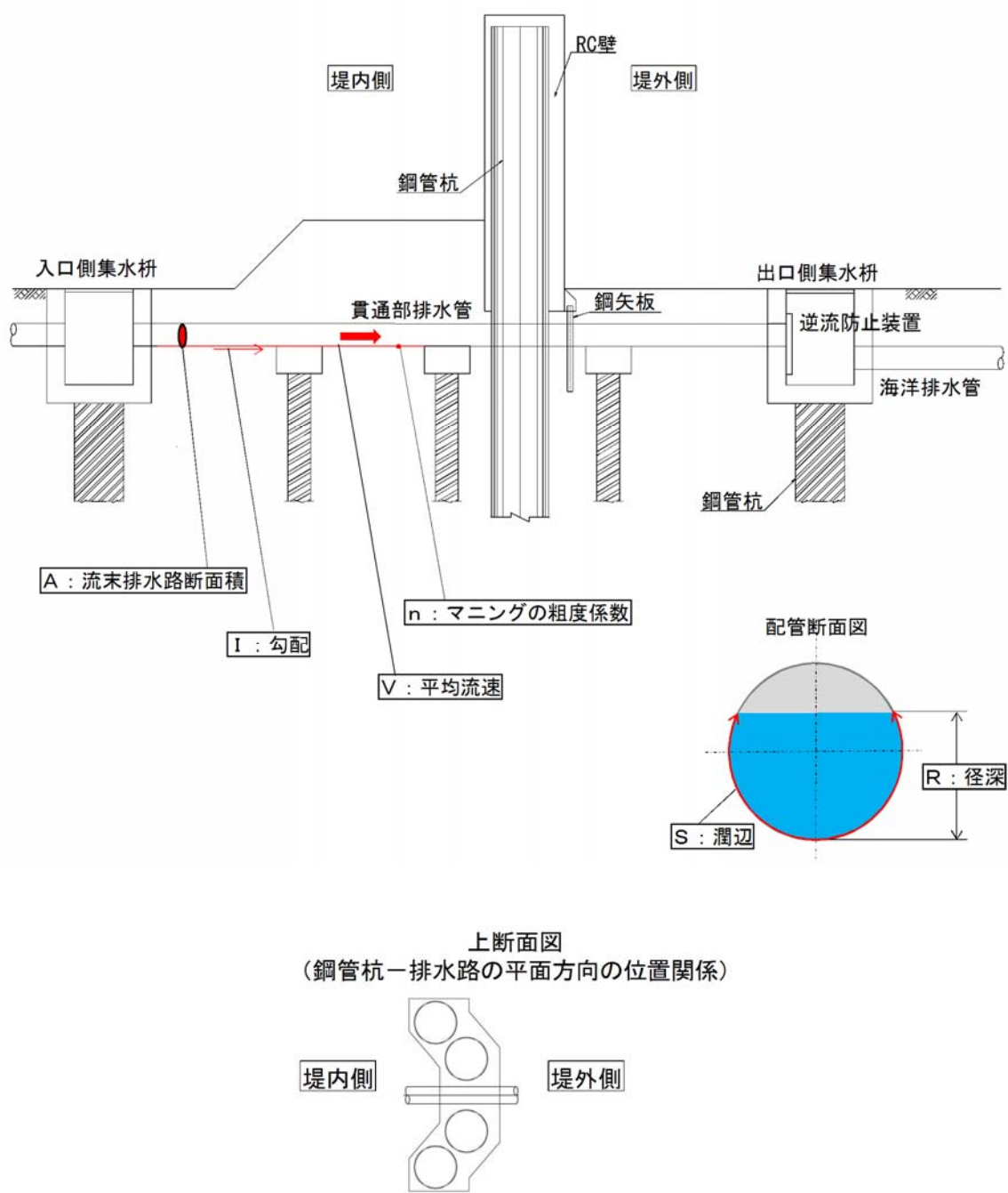
第 2 図 流末排水路構造（案）
