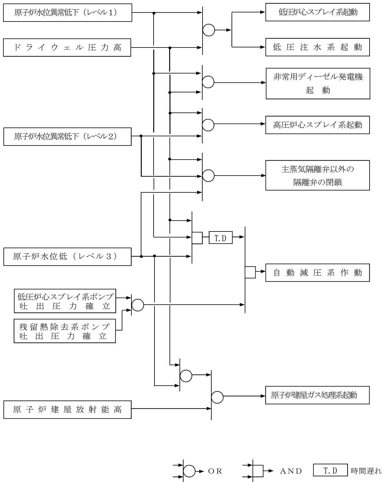
第 6.3-7 図 その他の主要な安全保護系機能説明図 (その 2)
