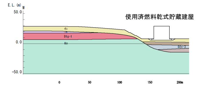
地質断面図
