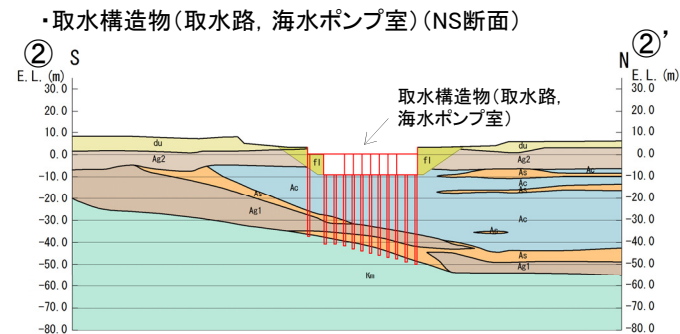
代表施設4(取水構造物(取水路, 海水ポンプ室))
