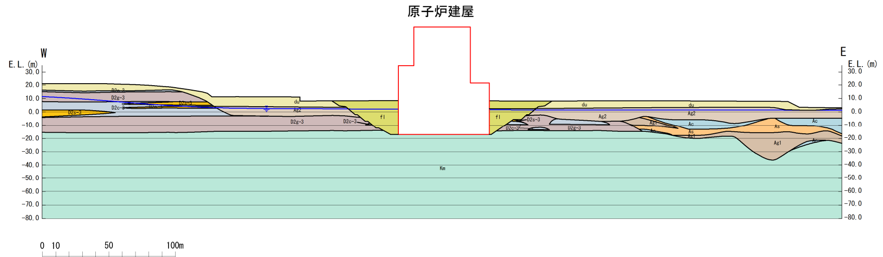
要素分割図のモデル化範囲
