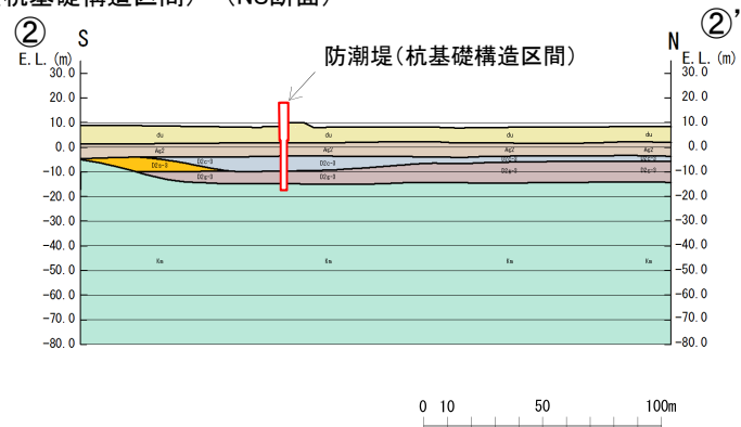
グループ③の地質断面図
