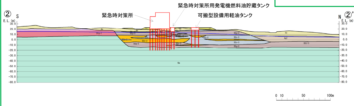
・緊急時対策所, 緊急時対策所用発電機燃料油貯蔵タンク, 可搬型設備用軽油タンク (NS断面)
