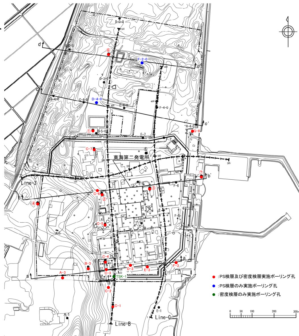
PS検層, 密度検層実施位置図
