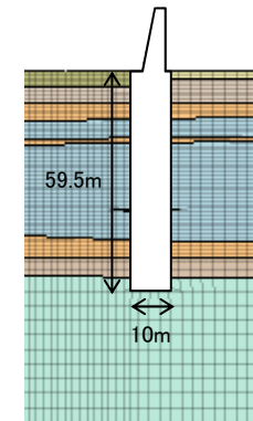
防潮堤 (地中連続壁基礎構造区間)
