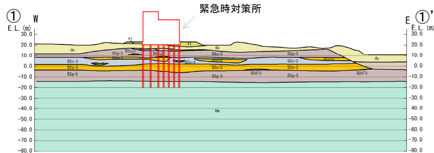
・緊急時対策所(EW断面)
