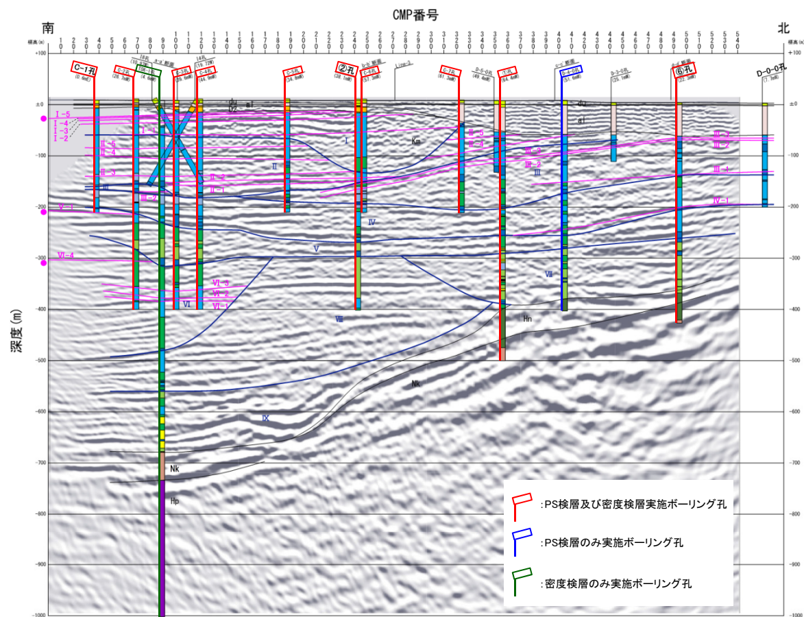
地質断面図 (Line-B)
