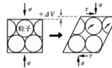
密な砂質土の体積膨張
