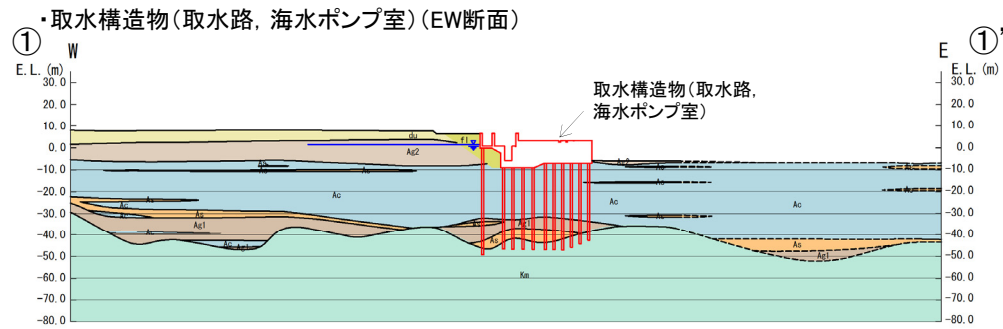
代表施設4(取水構造物(取水路, 海水ポンプ室))
