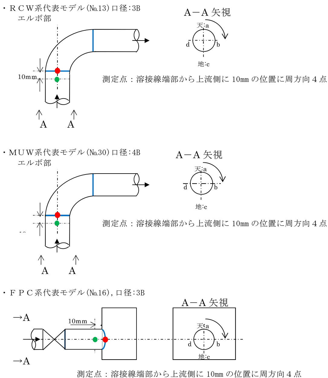
第1図 減肉測定位置図
