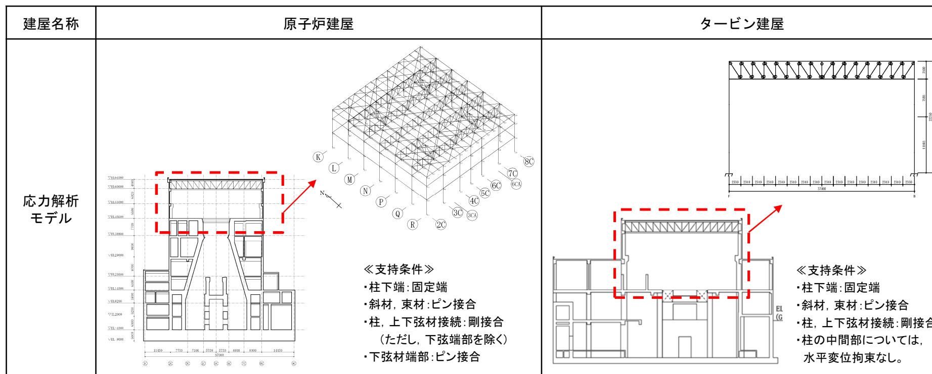
第2.2図 屋根トラスの解析モデル
