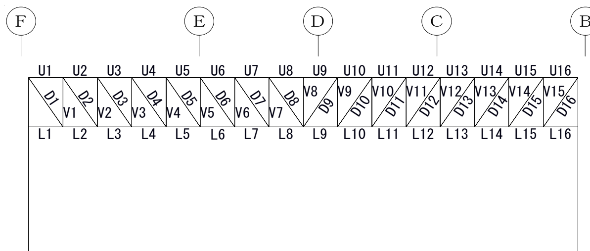
第2.4図 タービン建屋評価位置
