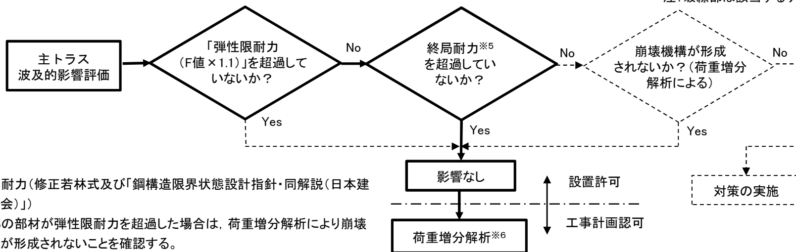
第2.1図 タービン建屋 主トラスの波及的影響評価フロー
