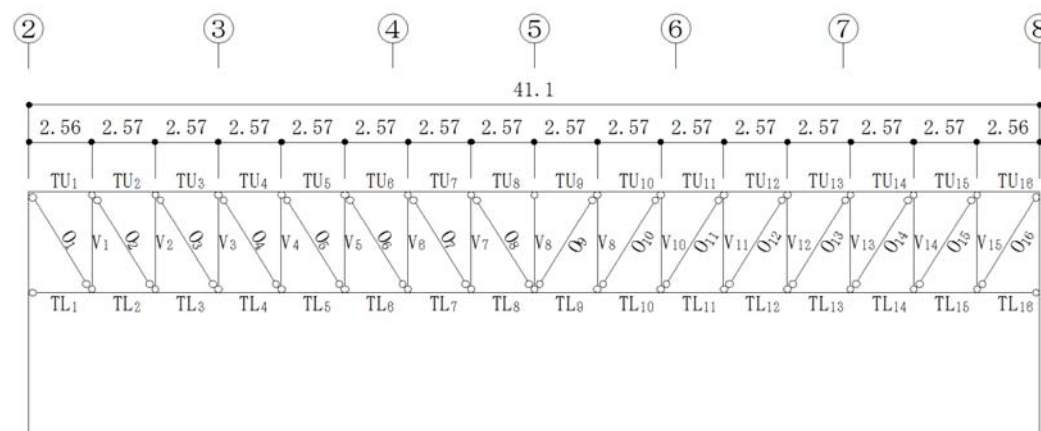
第2.3図 原子炉建屋評価位置
