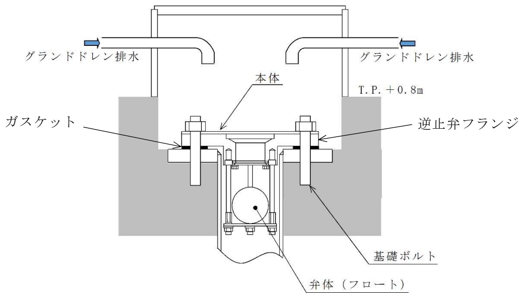
第 3.2-5 図 緊急用海水ポンプグラントドレン排出口逆止弁構造図
