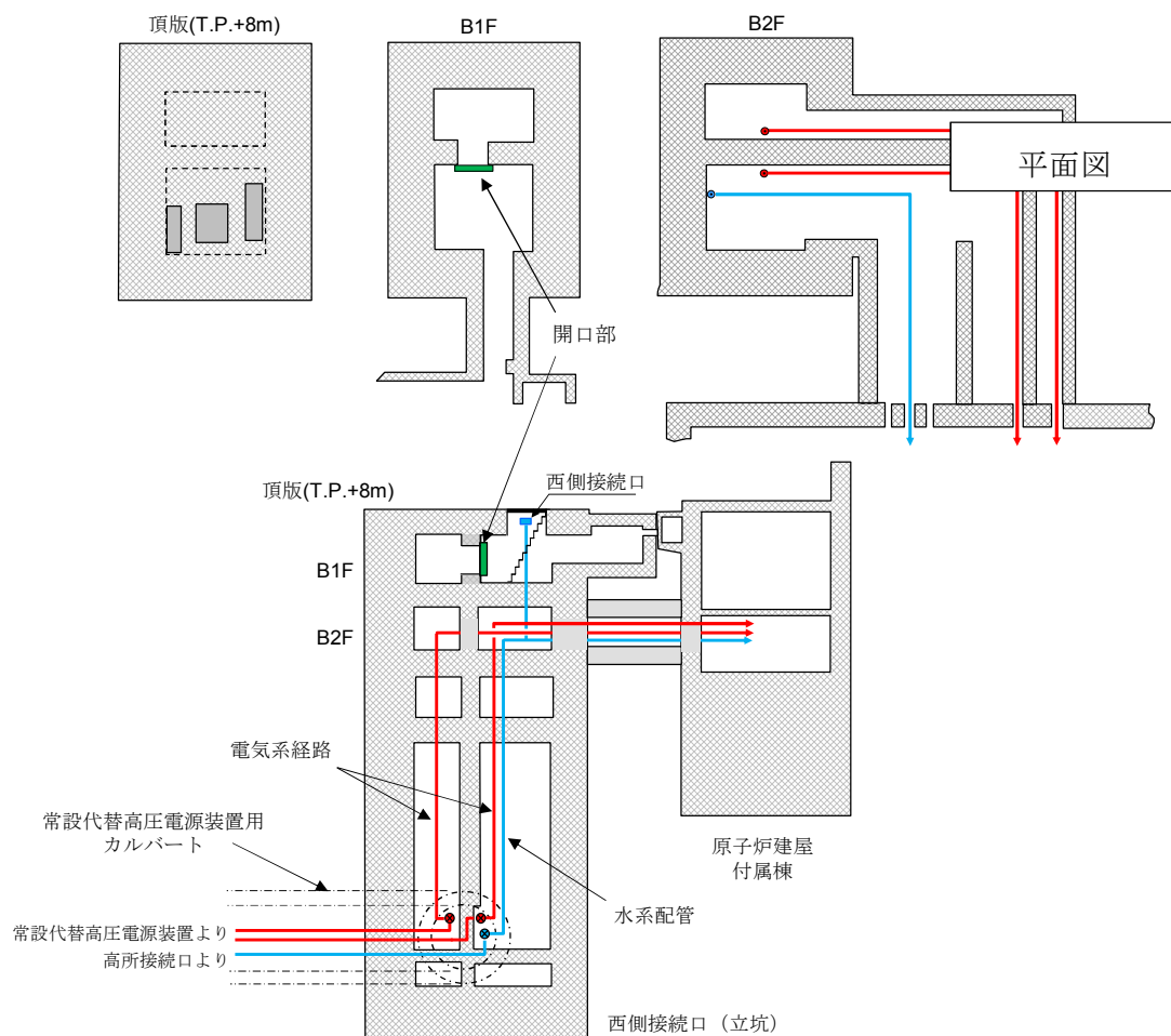
断面図
