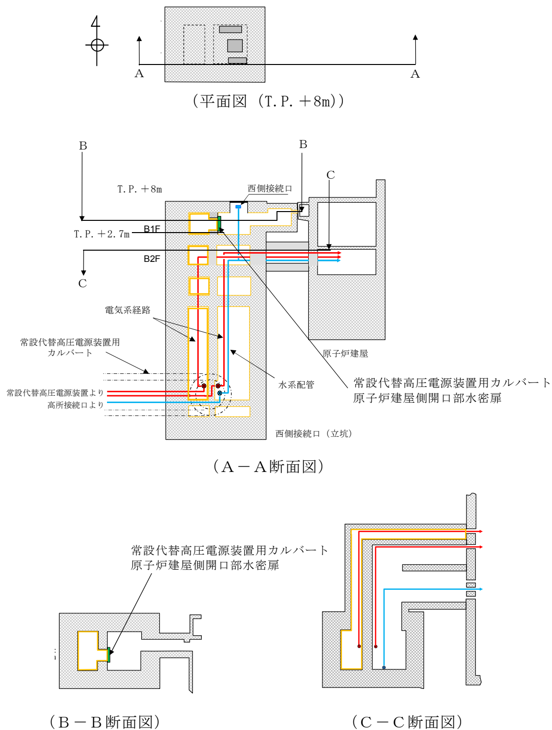
第 2.2.2-11 図 常設代替高圧電源装置用カルバート 原子炉建屋側開口部水密扉配置図
