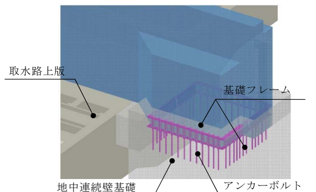
第 3.1-3 図 構造形式毎の防潮堤構造図 (1/4)
