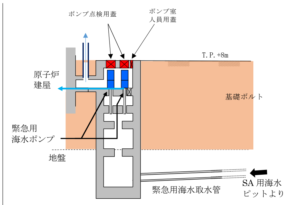
第 3.2-11 図 緊急用海水ポンプピット概略断面 図
