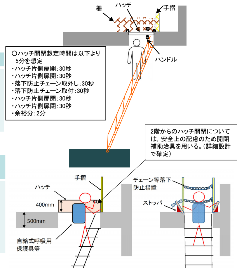
第1図 新設ハッチ部イメージ
