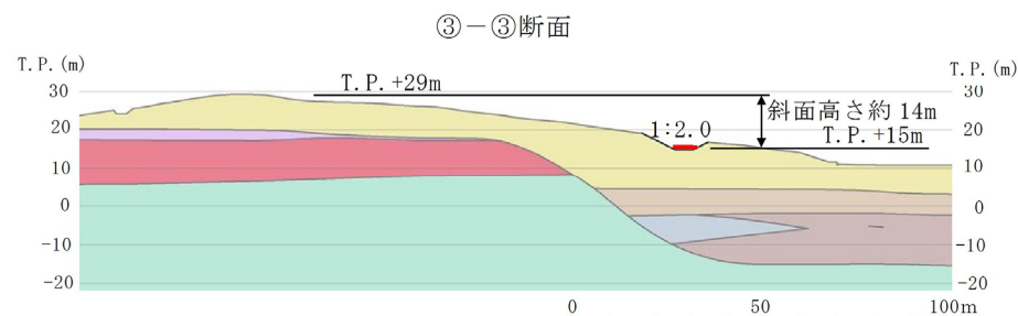
アクセスルートの周辺斜面の崩壊及び道路面のすべりに対する影響評価断面図
