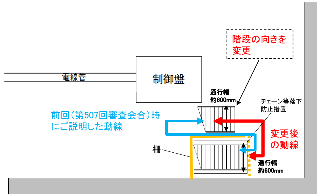
第2図 付属棟2階平面図
