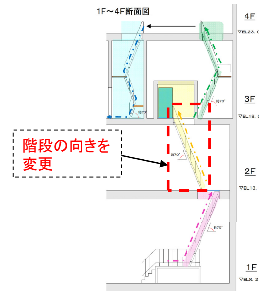
第4図 付属棟1階～4階断面図(変更後)
