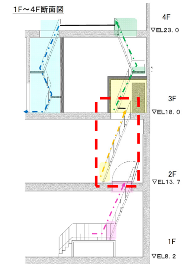
第3図 付属棟1階～4階断面図(変更前)
