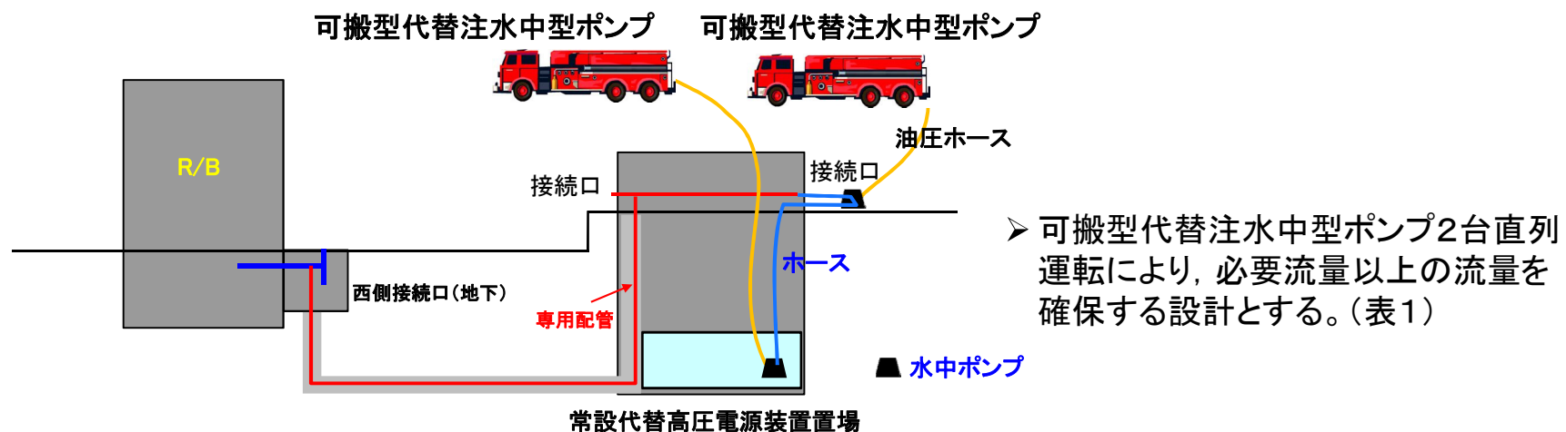
図2 原子炉への送水時の系統構成概要
